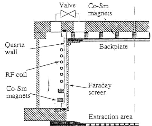
Рис. 3. Эскиз генератора RF плазмы, используемого для получения H в NBI ASDEX-U [13]
