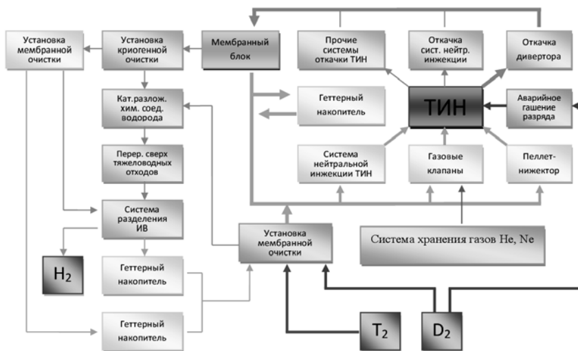
Рис. 1. Модернизированная схема функциональных элементов топливного цикла [1]. Толщина линий указывает на величину проходящего потока газов
