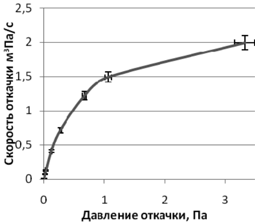
Рис. 4. Зависимость удельной скорости откачки трития ванадиевой мембраной площадью 1 м 2 от давления, при температуре атомизатора 2100 К и площади атомизатора 0,2 м [14]
