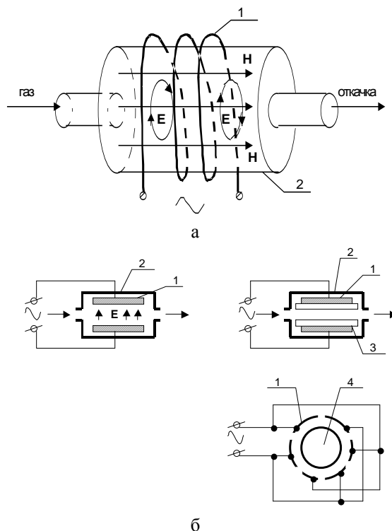
Рис. 2. Способы осуществления ВЧ-разряда низкого давления: а – индукционный разряд: 1 – индуктор, 2 – разрядная камера; б – емкостной разряд: 1 – электроды, 2 – разрядная камера, 3 – диэлектрические пластины, 4 – цилиндрическая кварцевая разрядная камера
