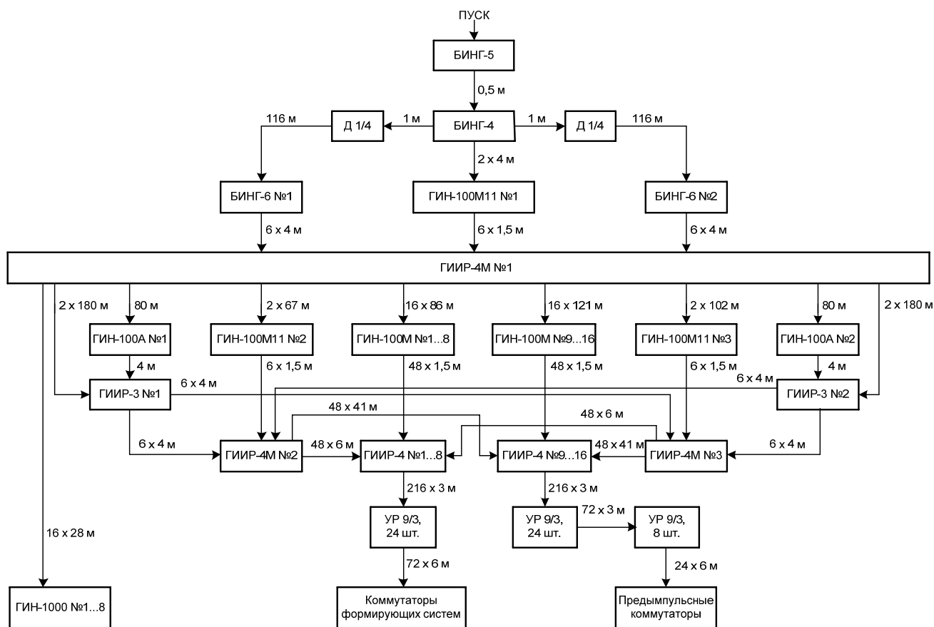
Рис. 3. Структурная схема системы синхронизации установки «Гамма-4»
