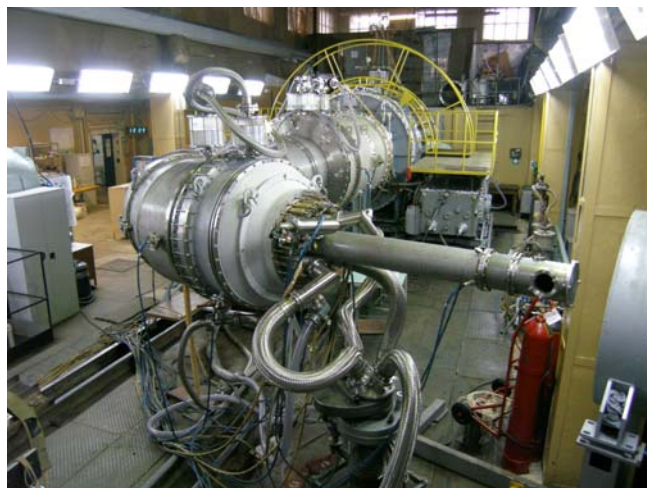
Рис. 1. Внешний вид ускорителя «Гамма-1»
