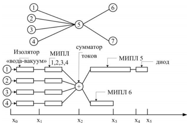
Рис. 3. Наверху – граф установки ГАММА-4, ниже – он же, но приведенный к единой пространственной переменной
