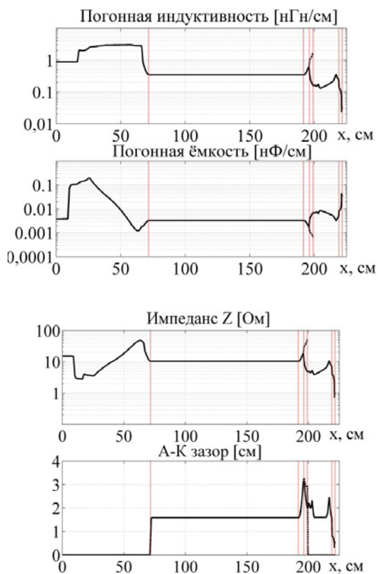
Рис. 4. Параметры одномерной модели установки. А-К зазор указан только для областей, в которых учитываются электронные утечки
