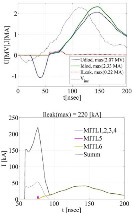
Рис. 5. Результаты расчетов работы установки ГАММА-4 с единой диодной нагрузкой, V_{inc} – напряжение в падающей волне
