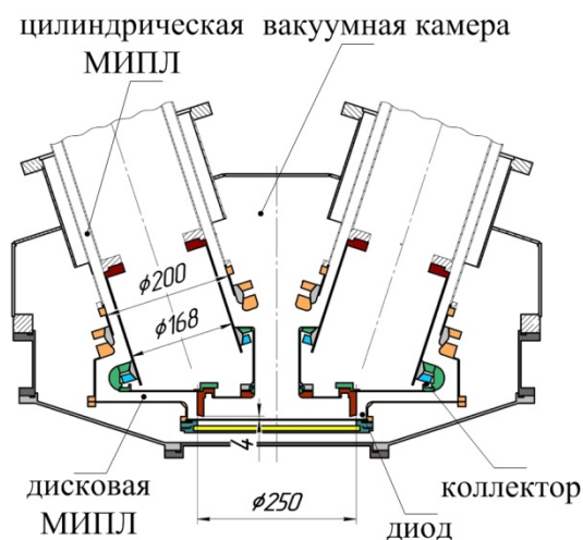
Рис. 1. Конструктивная схема объединения модулей на единую диодную нагрузку
