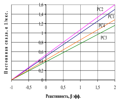
Рис. 10. Зависимость константы спада мгновенных нейтронов от реактивности для РС1 (РС со свинцом), РС2 (полая РС), РС3 (РС с МСБ1), РС4 (РС с МСБ2), измеренные при помощи БРИК/NMIS методики
