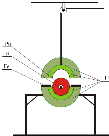
Рис. 1. Схема первого критмассового эксперимента (1949 г.)
