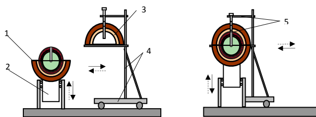
Рис. 8. Схематическое изображение ЭМС ФКБН-2М: 1 – НБ; 2 – стол, перемещаемый вертикально; 3 – ВБ; 4 – каретка, перемещаемая горизонтально; 5 – устройство загрузки центрального канала
