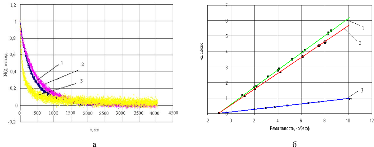
Рис. 9. Спады плотности мгновенных нейтронов во времени при \rho/\beta_{\text{эфф}} \approx -2 (а) и зависимости постоянной спада мгновенных нейтронов от реактивности (б) (1 – PC1; 2 – PC2; 3 – PC3)
