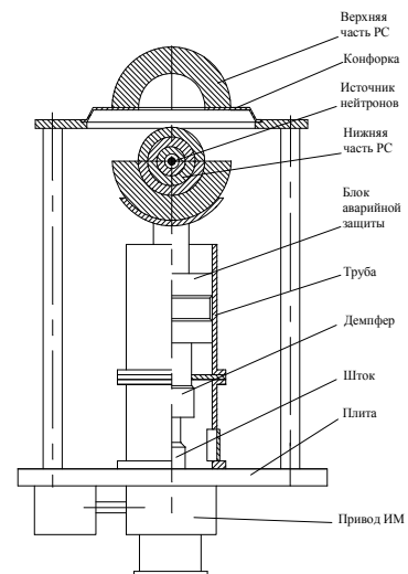
Рис. 4. Схема стэнда МСКС
