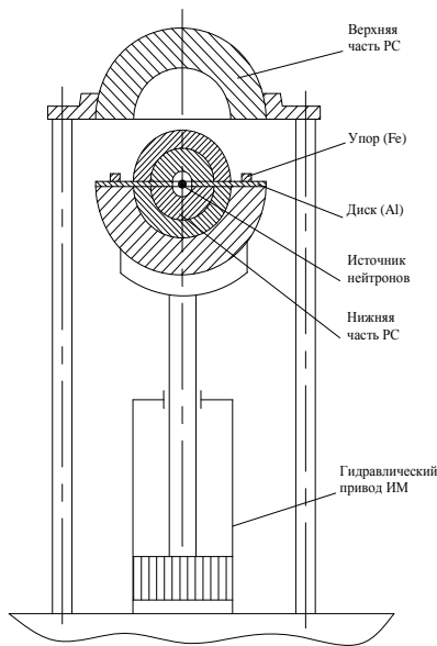
Рис. 2. Схема критического стэнда ФКБН (1950 г.)
