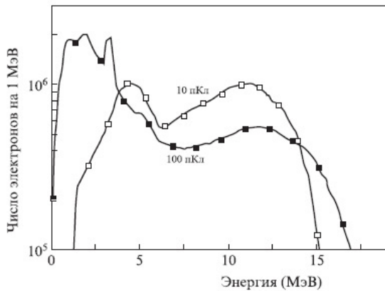
Рис. 3. Спектры электронов для разных начальных зарядов сгустка, формирующиеся в случае ускорения электронов лазерным импульсом круговой поляризации при \gamma_0 = 2 и a_0 = 5
