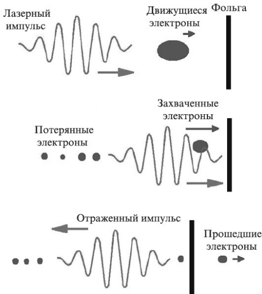
Рис. 1. Схема прямого лазерного ускорения электронного сгустка
