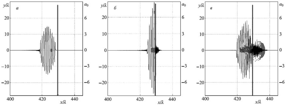
Рис. 2. Типичная картина PIC-моделирования прямого ускорения электронного сгустка линейно поляризованным лазерным импульсом (последовательно слева – направо). Наряду с распределением электронов показано распределение электрического поля лазерного импульса
