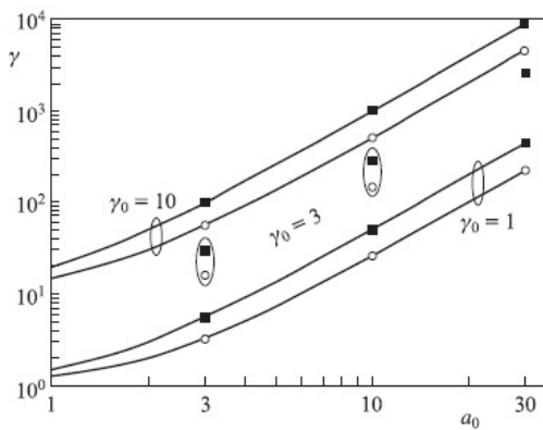
Рис. 4. Максимальная энергия электронов при вакуумном ускорении линейно (квадратик) и циркулярно (кружок) поляризованным лазерным импульсом в зависимости от амплитуды лазерного поля a_0 и начальной энергии пучка \gamma_0
