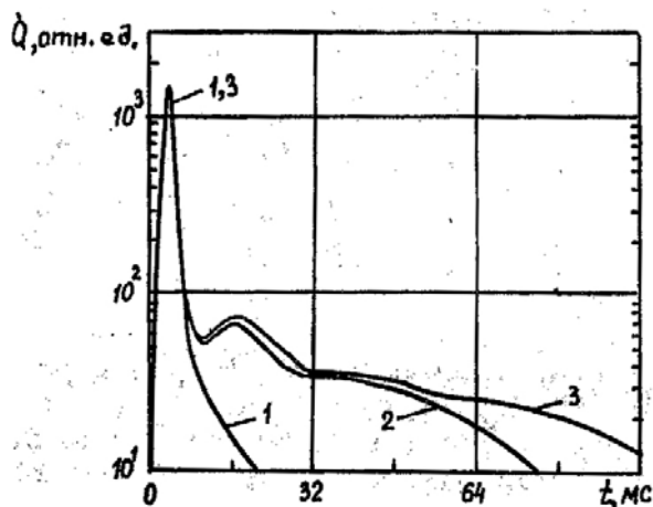
Рис. 6. Форма импульса делений в реакторе БИГР при различных режимах его работы: 1 – пролетный ( Q_0 = 10 Вт; \rho_0 = 0,083 \beta_{эф} ; Нис = 100 мм); 2 – пролетный ( Q_0 = 10 Вт; \rho_0 = 0,083 \beta_{эф} ; Нис = 400 мм); 3 – с остановкой ИС в АЗ при иницировании от ИНГ
