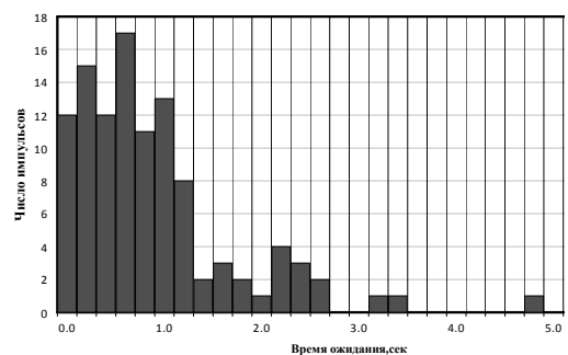
Рис. 12. Экспериментальная гистограмма зависимости чисел импульсов от времени ожидания для опытов серии из 115 пусков реактора БИР при \rho_p = 0,050\beta_{эф}
