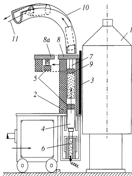
Рис. 8. Схема подвижной части установки: 1 – АЗ; 2 – блок замедлителя; 3 – экран из ВС_4 и Cd ; 4 – контейнер УХН; 5, 9 – охлаждаемый конвертор; 6 – система разгона; 7 – система торможения; 8, 8а – массивная подвижная плита; 10 – транспортный желоб; 11 – трос
