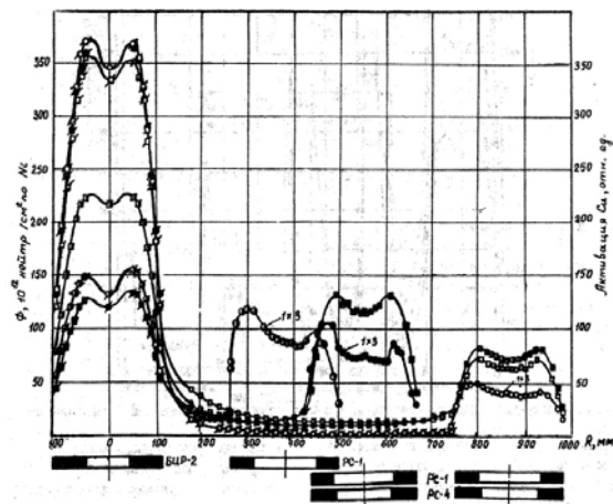
Рис. 4. Пространственные распределения флюенса нейтронов
