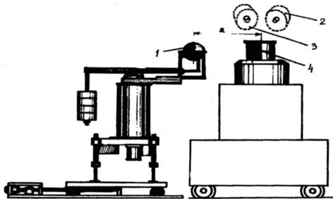
Рис. 3. Схема эксперимента: 1 – ПС, 2 и 3 – счетчики нейтронов, 4 – АЗ БИР
