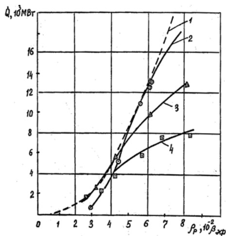
Рис. 5. Зависимость амплитуды импульса делений от реактивности для реактора БИР: 1 – иницирование от ИНГ при остановке ИС в АЗ; 2, 3, 4 – иницирование при начальной мощности в АЗ \approx 1 Вт и скорости пролета ИС через АЗ 28,8, 20,3 и 11,9 м/с, соответственно
