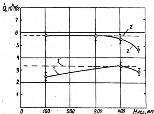
Рис. 7. Зависимость максимальной мощности в импульсе реактора БИГР от начального положения ИС в АЗ ( H_{ис} ): 1, 2 – пролетный режим ( Q_0 = 10 Вт ; \rho_0 = 0,06 \beta_{эф} и \rho_0 = 0,083 \beta_{эф} ); 1', 2' – режима с остановкой ИС в АЗ при инициировании от ИНГ
