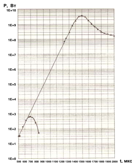
Рис. 10. Формы полномасштабного и оборванного с помощью БАЗ импульсов
