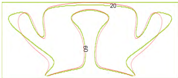
Рис. 2. Изолинии температуры на T = 20 лет
