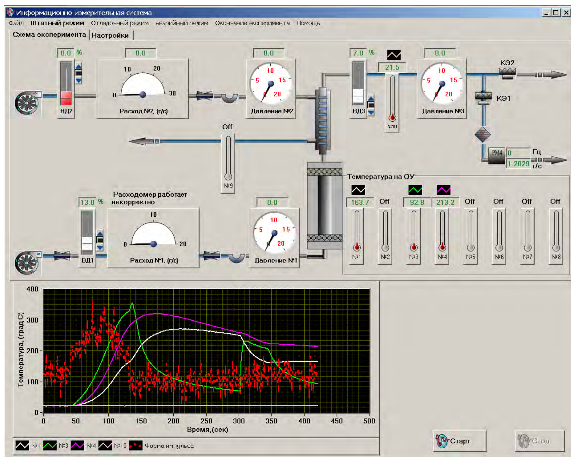
Рис. 4. Пример представления информации в виде мнемосхемы и графика
