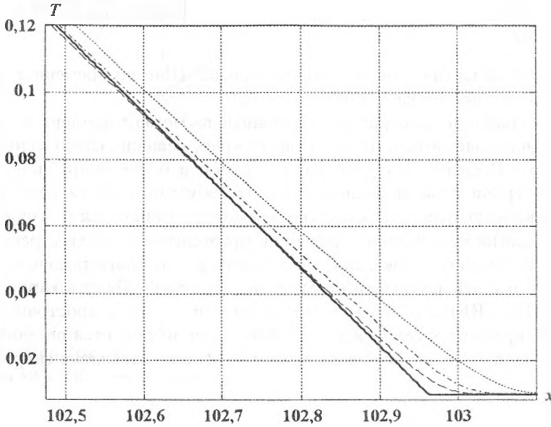
Рис. 4. Тест 2. Профиль T(x) на момент времени ct = 14\,400 (в окрестности фронта температурной волны в укрупненном масштабе), рассчитанный по St-схеме, в сравнении с точным решением: \cdots\cdots — сетка 360 \times 24 ; \cdots - \cdots — сетка 720 \times 24 ; - \cdot - \cdot - — сетка 1\,440 \times 24 ; — — точное решение
