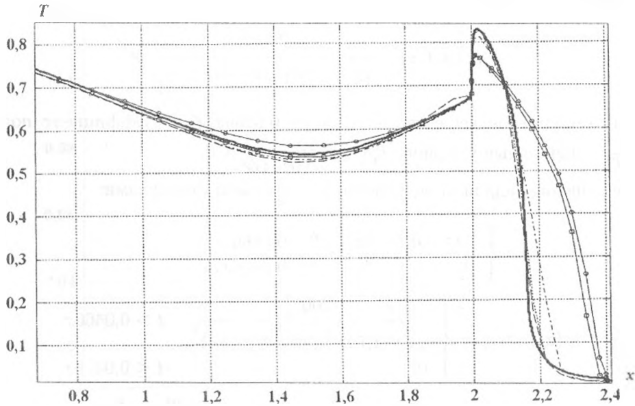
Рис. 1. Тест 1. Профиль T(x) на момент времени ct = 9 на сетке 56 \times 12 : —○— St-схема; ..... MDS n -схема; —□— DD\St-схема; --- REED-схема; - · - · DDAD-схема; — — — точное решение
