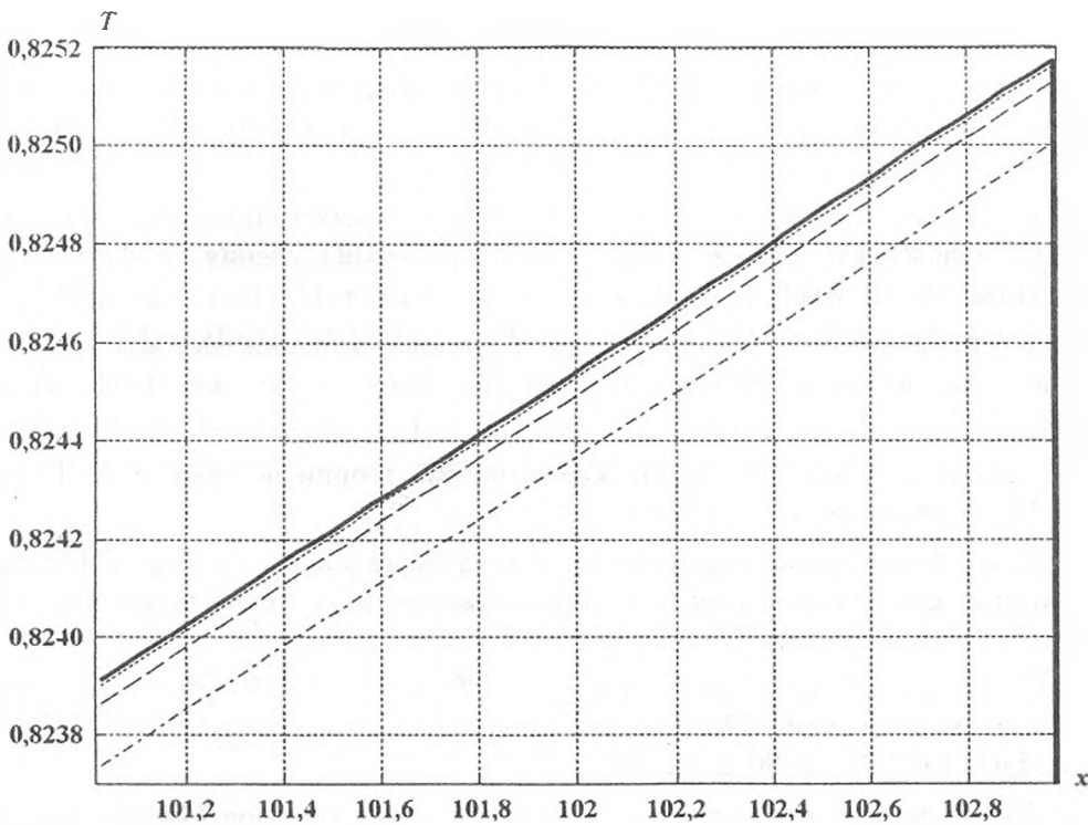
Рис. 6. Тест 3. Профиль T(x) слева от разрыва в области 1 на момент времени ct = 30 (в укрупненном масштабе), рассчитанный по St-схеме, в сравнении с точным решением: - · - · - сетка 80 \times 60 ; - - - - сетка 80 \times 120 ; ······ — сетка 80 \times 240 ; — — — — точное решение
