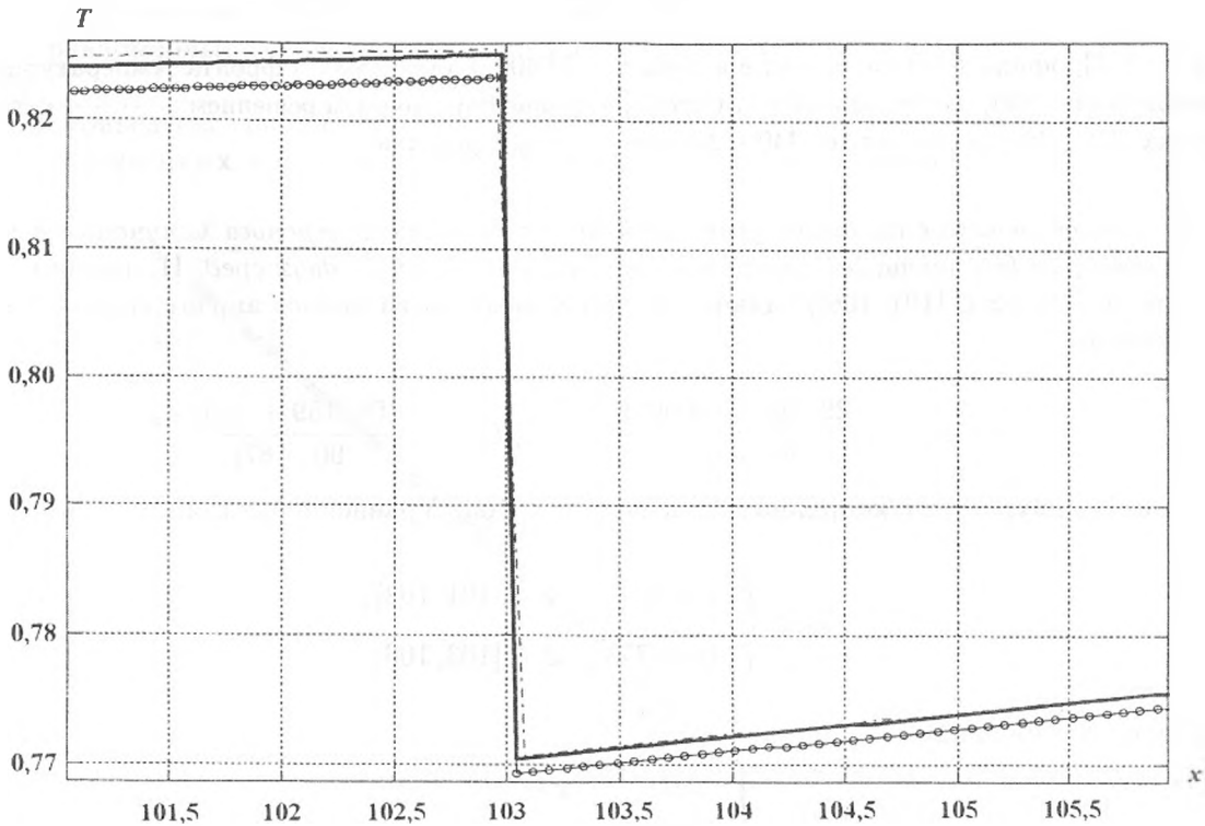
Рис. 5. Тест 3. Профиль T(x) на момент времени ct = 30 (результаты по схемам St, DD\St, REED, MDS_n практически совпадают): - - - DDAD-схема, сетка 80 \times 12 ; -o- DD\St-схема, сетка 80 \times 12 ; — — точное решение
