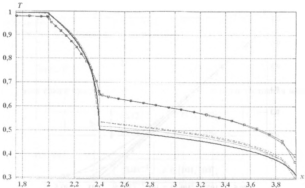
Рис. 2. Тест 1. Профиль T(x) на момент времени ct = 400 на сетке 56 \times 12 (области 2 и 3): —○— St-схема; ..... MDS n -схема; —□— DD\St-схема; --- REED-схема; - · - · DDAD-схема; — — — точное решение
