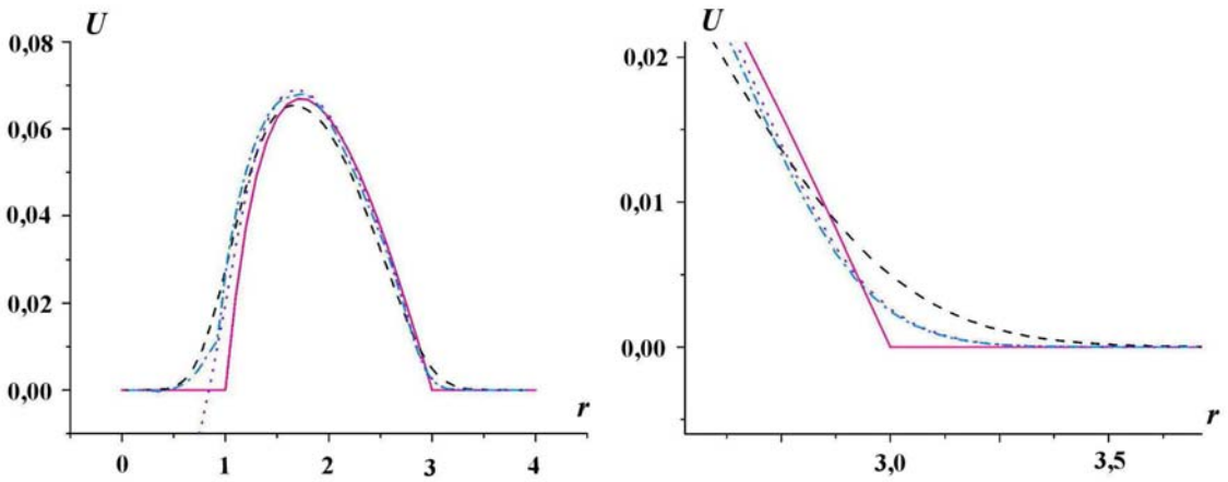
Рис. 8. Тест 5. Профили плотности энергии излучения в сечении под углом 45^\circ на момент времени t = 2 : - - - - по схеме 1; \cdots — по схеме 2; - · - · - по схеме 3; — — — — аналитическое решение
