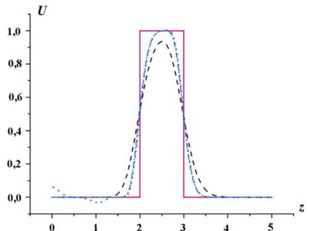
Рис. 2. Тест 1. Профили плотности энергии излучения на момент времени t = 1 : — — — по схеме 1; ··· — по схеме 2; - · - · по схеме 3; — — — аналитическое решение
