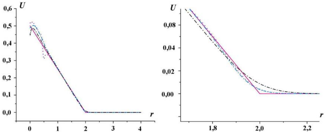
Рис. 7. Тест 5. Профили плотности энергии излучения в сечении под углом 45^\circ на момент времени t = 1 : - - - - по схеме 1; \cdots — по схеме 2; - · - · - по схеме 3; — — — — аналитическое решение
