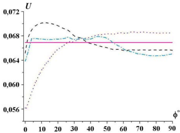
Рис. 9. Тест 5. Зависимость плотности энергии излучения от угла при r = 1,7 ; t = 2 : - - - - по схеме 1; \cdots — по схеме 2; - · - · - по схеме 3; — — — — аналитическое решение
