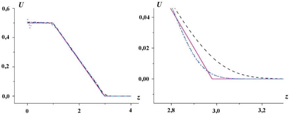
Рис. 5. Тест 3. Профили плотности энергии излучения на момент времени t = 2 : — — — по схеме 1; ... — по схеме 2; - · - · - по схеме 3; — — — — аналитическое решение
