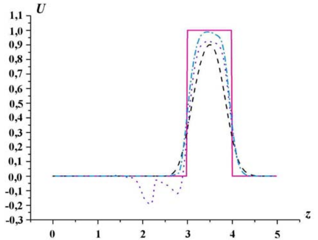
Рис. 4. Тест 2. Профили плотности энергии излучения на момент времени t = 1,4 : — — — по схеме 1; ··· — по схеме 2; - · - · — по схеме 3; — — — аналитическое решение
