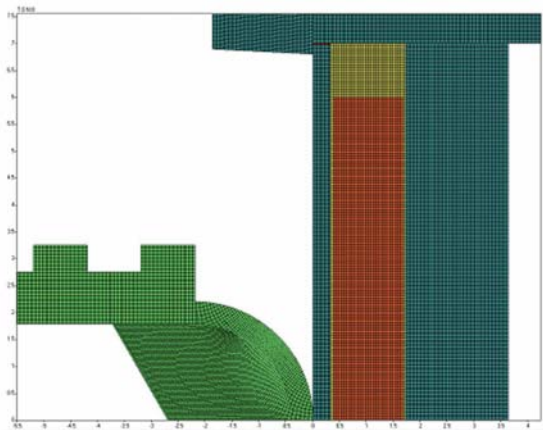
Рис. 7. Фрагмент пространственной сетки в расчете по методике Д
