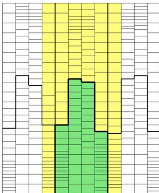
Рис. 3. Фрагмент расчетной сетки со счетными ячейками и ячейками наложения для одного процессора
