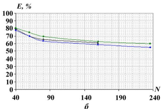
Рис. 11. Зависимости времени расчетов (а) и эффективности распараллеливания (б) от количества процессоров для задачи 2: —▲— — одномерная декомпозиция; —■— — двумерная декомпозиция; —◆— — комбинированная декомпозиция
