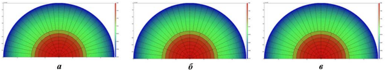
Рис. 9. Расчетное поле температур на конечный момент времени стационарной двухобластной задачи с функцией источника: а — одномерная декомпозиция; б — двумерная декомпозиция; в — комбинированная двумерная декомпозиция
