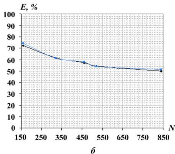
Рис. 10. Зависимости времени расчетов (а) и эффективности распараллеливания (б) от количества процессоров для задачи 1: —◆— — одномерная декомпозиция; —●— — двумерная декомпозиция
