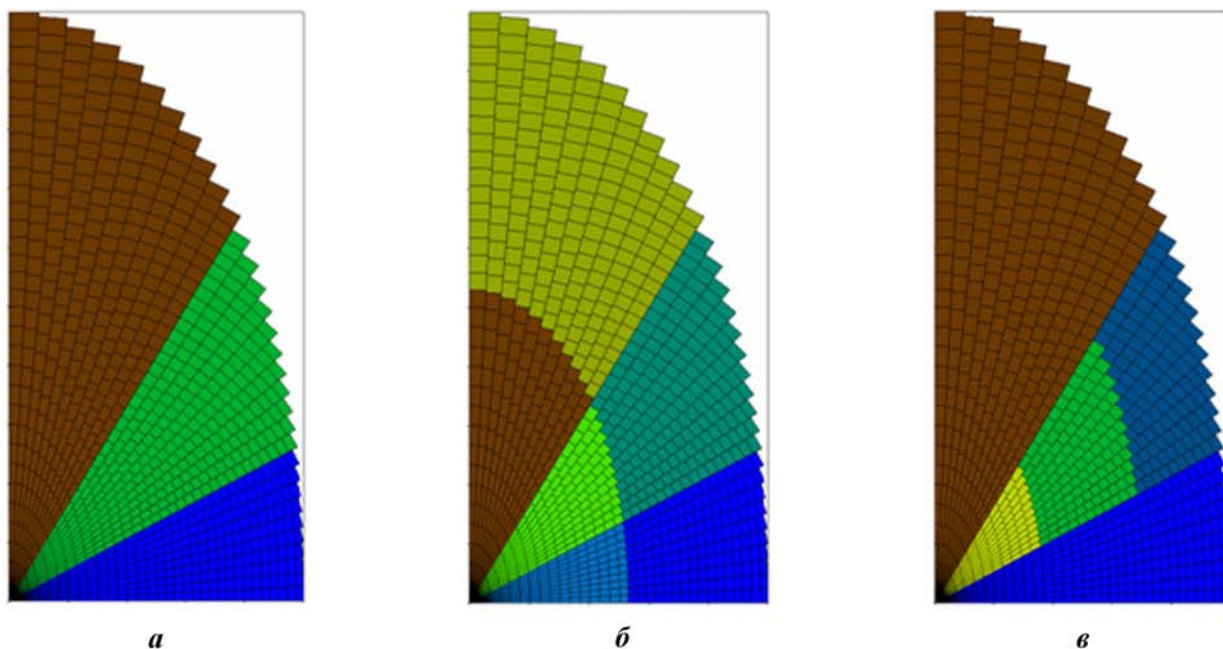
Рис. 5. Декомпозиции расчетной сетки: a — одномерная; b — двумерная; в — комбинированная двумерная
