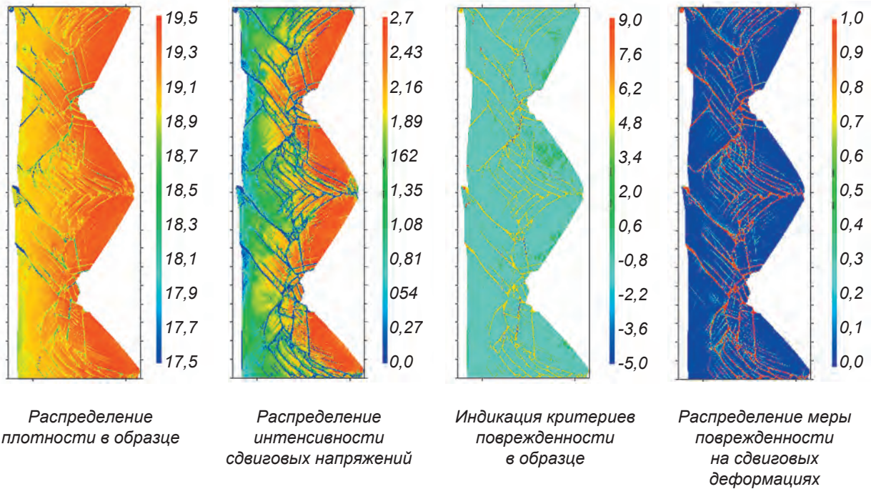
Численное моделирование повреждения материала при интенсивном ударно-волновом нагружении. Методика ТИМ-2D
