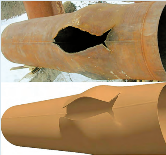
Состояние трубы после опыта
