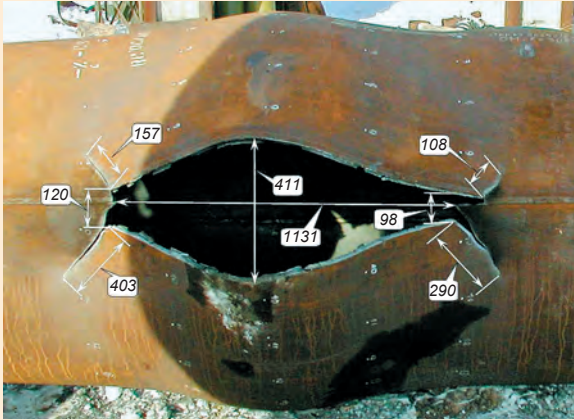
Зона разрушения (размеры указаны в мм)
