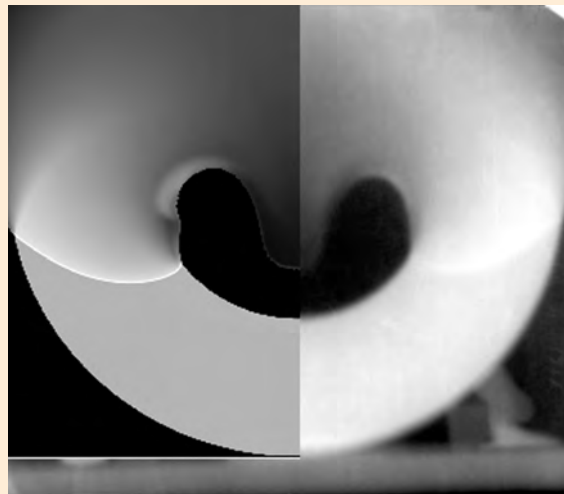
Распространение детонации в кольцевой шашке. Поле плотности: эксперимент (справа); расчет по программ ЛЭГАК-3D (слева)
