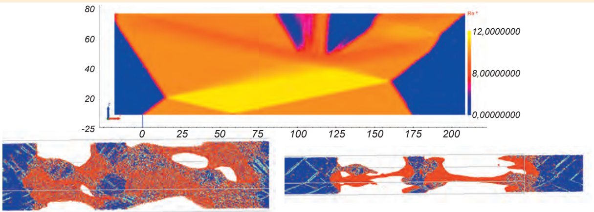
Процесс развития откола и визуализация частиц
