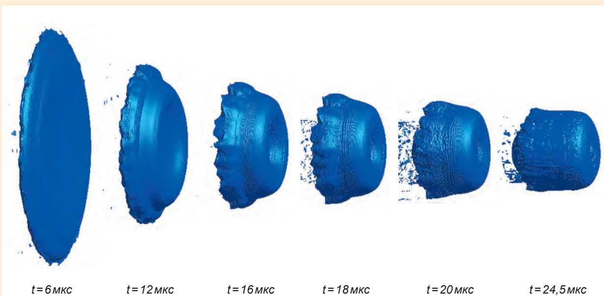
Динамика формирования ПЭ из тантала, полученная в расчете по программ ЛЭГАК-3D
