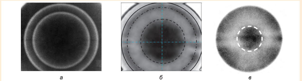
Рентгенограммы в эксперименте с дейтерием: а – устройство в исходном состоянии; б – t = 21,08 мкс; в – t = 24,26 мкс (момент максимального сжатия). Пунктиром показаны границы оболочек, полученные в результате обработки рентгенограмм
