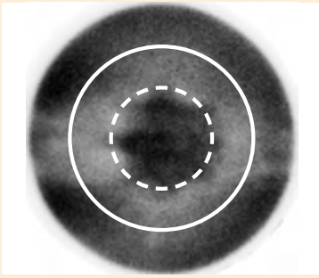
Рентгенограмма полости со сжатым гелием. Белым пунктиром и белой линией показаны результаты функциональной обработки рентгеновского изображения полости со сжатым гелием и радиуса волны сжатия в стальной оболочке на момент максимального сжатия газа
