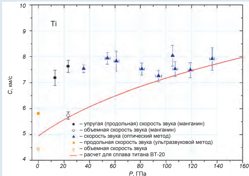
Зависимость скорости звука в титане от давления
