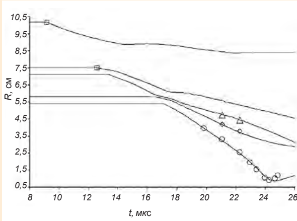
R(t) диаграммы движения оболочек в эксперименте с дейтерием, времена отсчитываются от начала детонации заряда ВВ: \square – электроконтактные измерения движения УВ при газодинамическом исследовании устройства; результаты рентгенографирования: \triangle – внутренняя граница первого каскада; \diamond – внешняя граница второго каскада; \circ – внутренняя граница второго каскада
