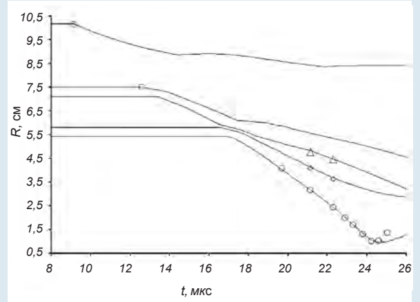
R(t) диаграммы движения границ оболочек в эксперименте с газообразным гелием ( P_0 = 167 атм; T_0 = 27 °С): \square – электроконтактные измерения движения УВ при газодинамическом исследовании устройства; результаты рентгенографирования: \triangle – внутренняя граница первого каскада; \diamond – внешняя граница второго каскада; \circ – внутренняя граница второго каскада
