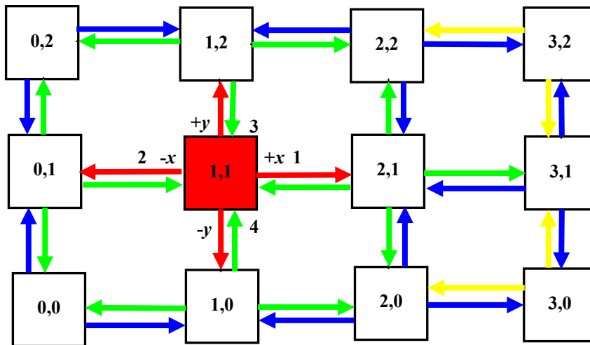
Рис. 1. Механизм первоначальной инициализации ВС
