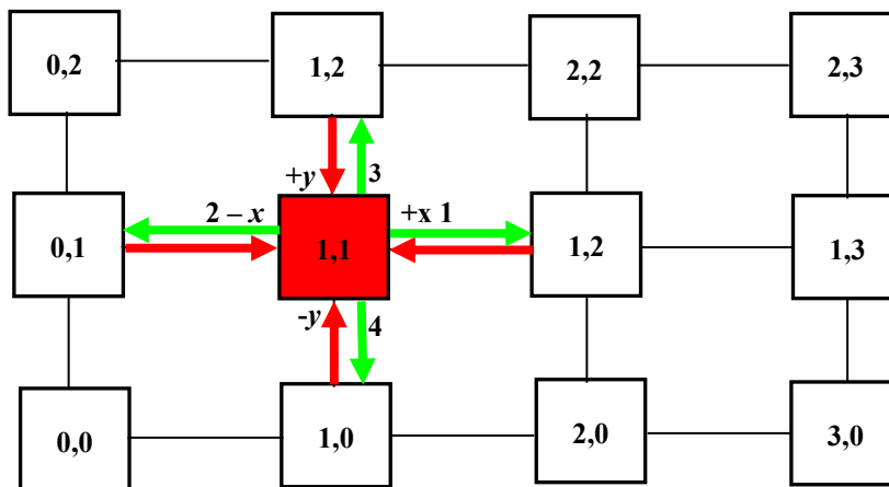
Рис. 2. Механизм инициализации повторно включаемых ВМ
