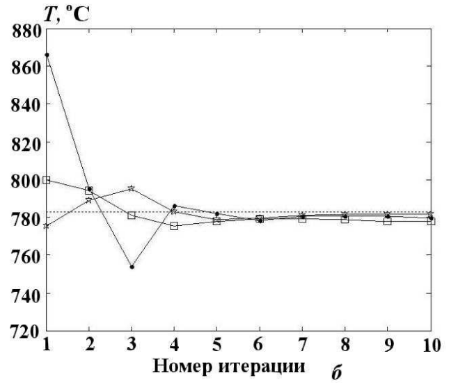
Рис. 2. Средняя температура топлива на половине высоты активной зоны при моделировании стационарной марковской цепи с использованием двух вариантов определения начального поколения: a — вариант 1; b — вариант 2; —*— — L = 5 ; —□— — L = 20 ; —●— — L = 100 ; ..... — эталон
