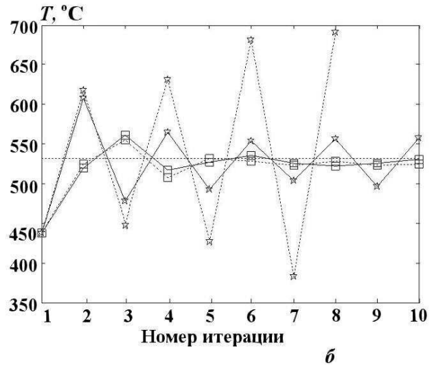
Рис. 3. Расчетная температура топлива в нижней части ТВС 1: a — L = 5 ; b — L = 100 ; ...*... — вариант 1, \varepsilon = 0 ; ...□... — вариант 1, \varepsilon = 1/2 ; —●— — вариант 2, \varepsilon = 0 ; —□— — вариант 2, \varepsilon = 1/2 ; ..... — эталон
