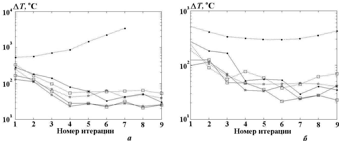
Рис. 1. Значения максимального отклонения температуры на последующих итерациях при моделировании стационарной марковской цепи с использованием двух вариантов определения начального поколения: a — вариант 1; б — вариант 2; —*—*— \varepsilon = 1/2, L = 5 ; —□—□— \varepsilon = 1/2, L = 20 ; —●—●— \varepsilon = 1/2, L = 100 ; ...*... \varepsilon = 0, L = 5 ; ...□... \varepsilon = 0, L = 20 ; ...●... \varepsilon = 0, L = 100
