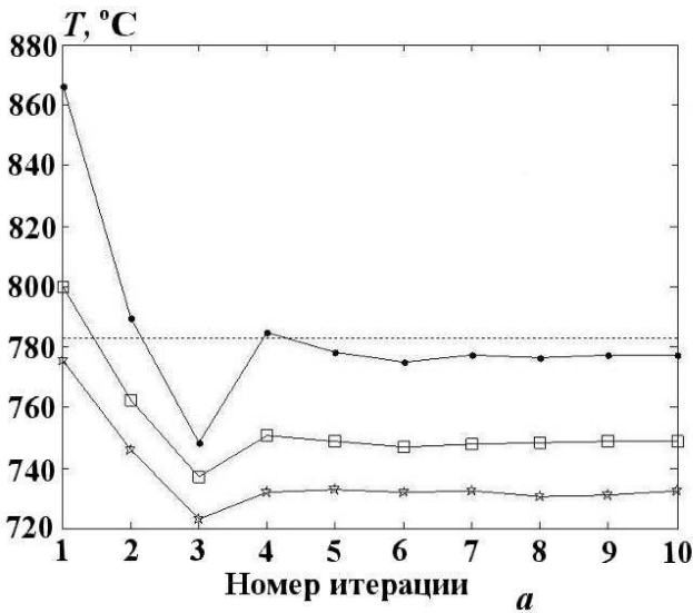
Рис. 2. Средняя температура топлива на половине высоты активной зоны при моделировании стационарной марковской цепи с использованием двух вариантов определения начального поколения: a — вариант 1; b — вариант 2; —*— — L = 5 ; —□— — L = 20 ; —●— — L = 100 ; ..... — эталон
