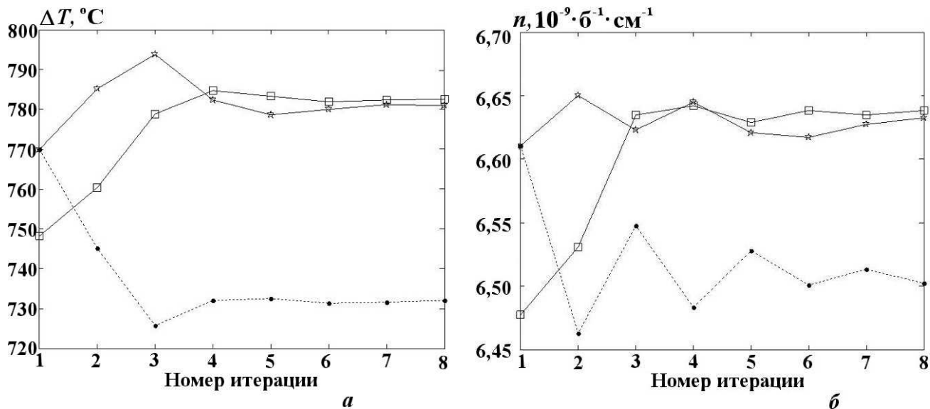
Рис. 6. Расчетные зависимости, полученные на половине высоты активной зоны при моделировании нестационарной марковской цепи с L = 5 : a — средняя температура топлива; б — средняя равновесная концентрация ^{135}\text{Xe} в центральной ТВС; —□— вариант 2, M/N = \text{const} ; —*— вариант 2, M = \text{const} ; ---•--- вариант 1, M = \text{const}
