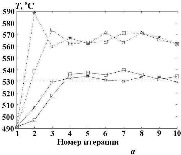
Рис. 3. Расчетная температура топлива в нижней части ТВС 1: a — L = 5 ; b — L = 100 ; ...*... — вариант 1, \varepsilon = 0 ; ...□... — вариант 1, \varepsilon = 1/2 ; —●— — вариант 2, \varepsilon = 0 ; —□— — вариант 2, \varepsilon = 1/2 ; ..... — эталон
