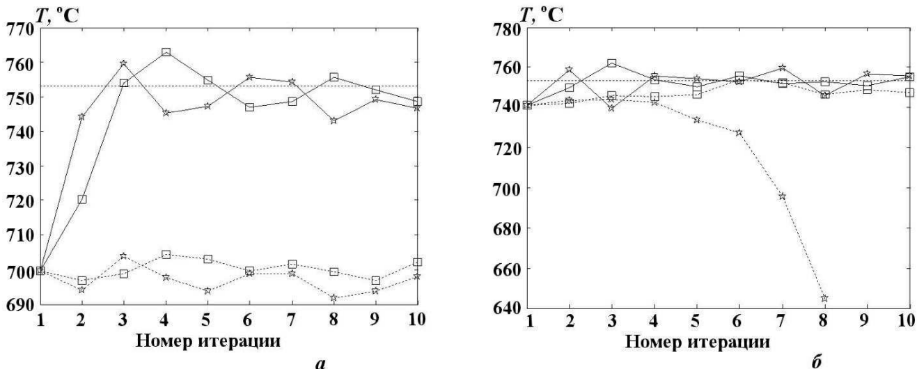
Рис. 4. Расчетная температура топлива в центре ТВС 82: a — L = 5 ; b — L = 100 ; \cdots* — вариант 1, \varepsilon = 0 ; \cdots\square\cdots — вариант 1, \varepsilon = 1/2 ; \text{—}* — вариант 2, \varepsilon = 0 ; \text{—}\square\text{—} — вариант 2, \varepsilon = 1/2 ; \cdots\cdots — эталон
