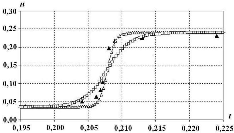
Рис. 9. Зависимости массовой скорости КГ образца — опорная пластина от времени в расчетах с физической вязкостью и без нее на сетке 2n : ▲ — эксперимент; ---△ — \eta = 0 ; □ — \eta = 0,01
