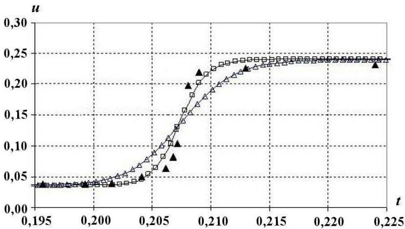
Рис. 10. Зависимости массовой скорости КГ образца — опорная пластина от времени в расчетах с физической вязкостью и без нее на сетке n : ▲ — эксперимент; ---△ — \eta = 0,01 ; □ — \eta = 0
