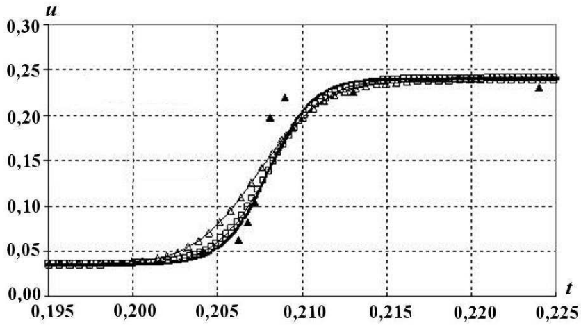
Рис. 8. Зависимости массовой скорости КГ образца — опорная пластина от времени в расчетах на сходимость с \eta = 0,01 без линейной вязкости: ▲ — эксперимент; — — расчет на сетке 4n ; □ — расчет на сетке 2n ; ---△ — расчет на сетке n
