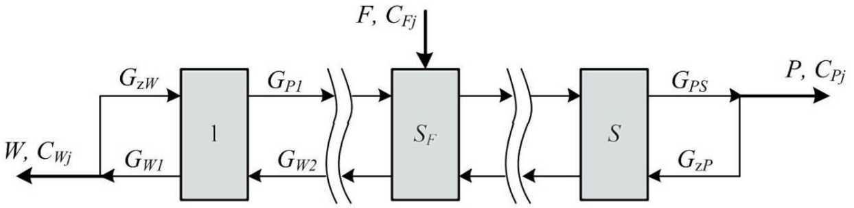
Рис. 1. Разделительный каскад
