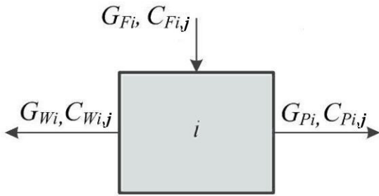
Рис. 2. Разделительная ступень
