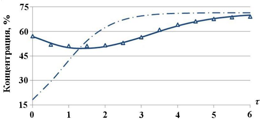
Рис. 5. Изменение концентрации ^{84}\text{Kr} в потоке тяжелой фракции каскада во времени: — — предлагаемая модель, начальное состояние 1; - - - предлагаемая модель, начальное состояние 2; \Delta — модель [6]
