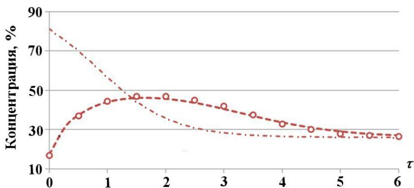
Рис. 6. Изменение концентрации ^{86}\text{Kr} в потоке тяжелой фракции каскада во времени: - - - предлагаемая модель, начальное состояние 1; - - - предлагаемая модель, начальное состояние 2; \circ — модель [6]
