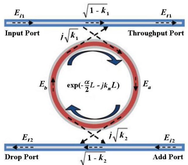
Рис. 4. Схема оптического кольцевого резонатора из [39]
