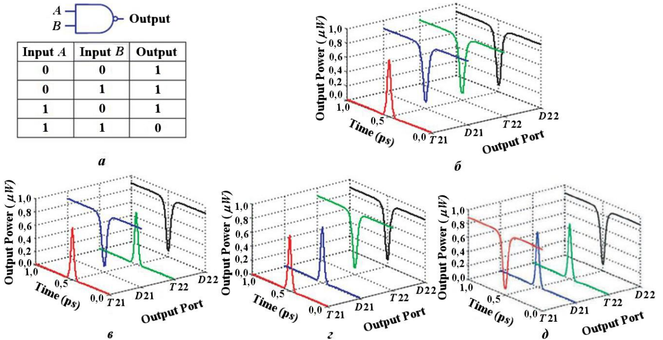
Рис. 6. Таблица истинности NAND (а) и выходные сигналы при входных сигналах A и B : "00" (б); "01" (в); "10" (г); "11" (д)
