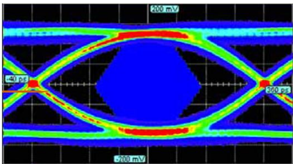
Рис. 3. Глаз-диаграмма выходных оптических сигналов
