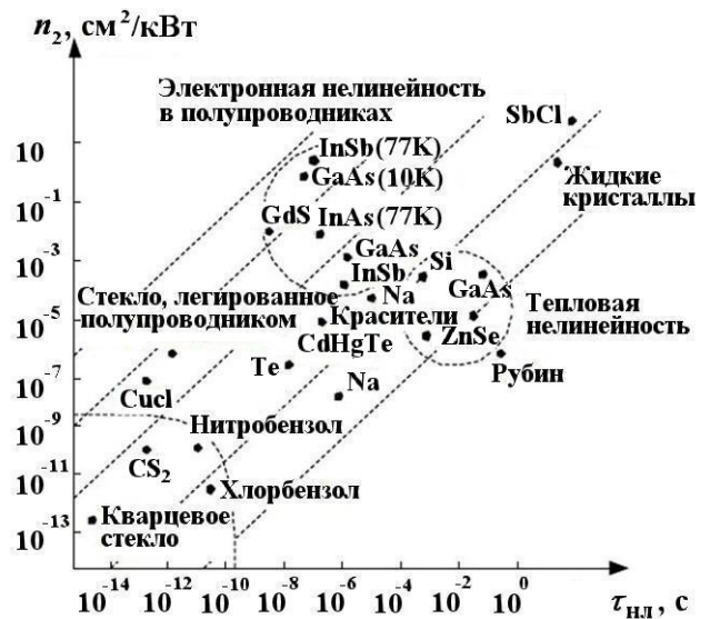
Рис. 1. Зависимости нелинейного показателя преломления от времени релаксации из [8]
