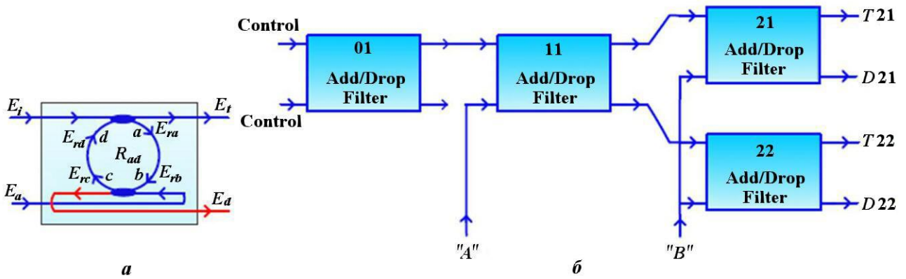
Рис. 5. Схемы МКР (а) и ОЛЭ NAND (б) из [31]
