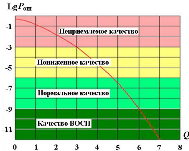
Рис. 2. Зависимость вероятности ошибки от Q -фактора
