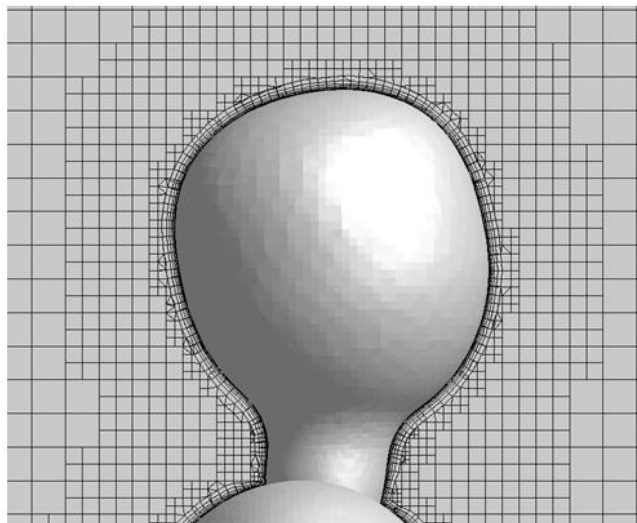
Рис. 5. Сечение расчетной сетки в области головы модели
