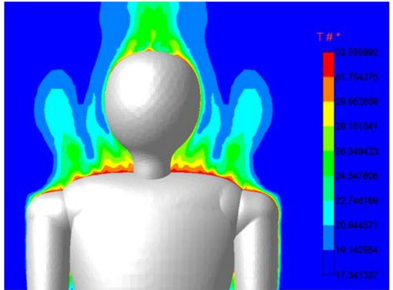
Рис. 6. Распределение температуры в окрестности модели человека
