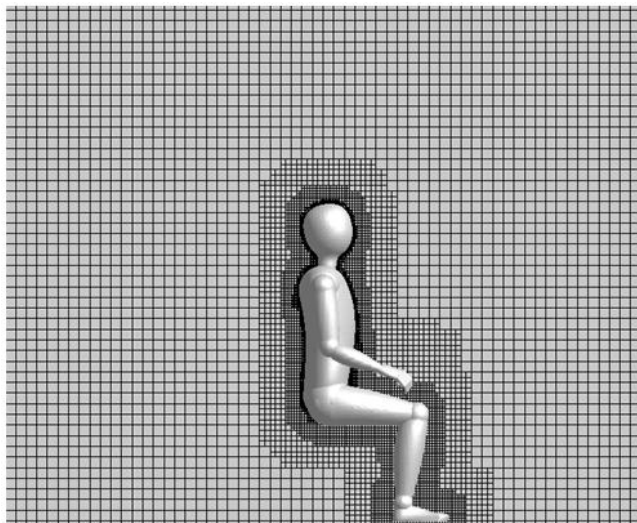
Рис. 4. Сечение области расчета модели человека
