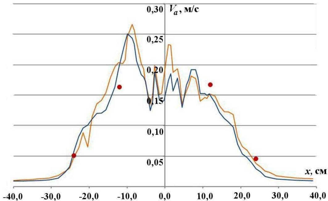
Рис. 8. Распределение скорости потока воздуха на горизонтальной прямой в 3 см над головой: ● — эксперимент; — ЛОГОС без использования TCM; — ЛОГОС с использованием TCM
