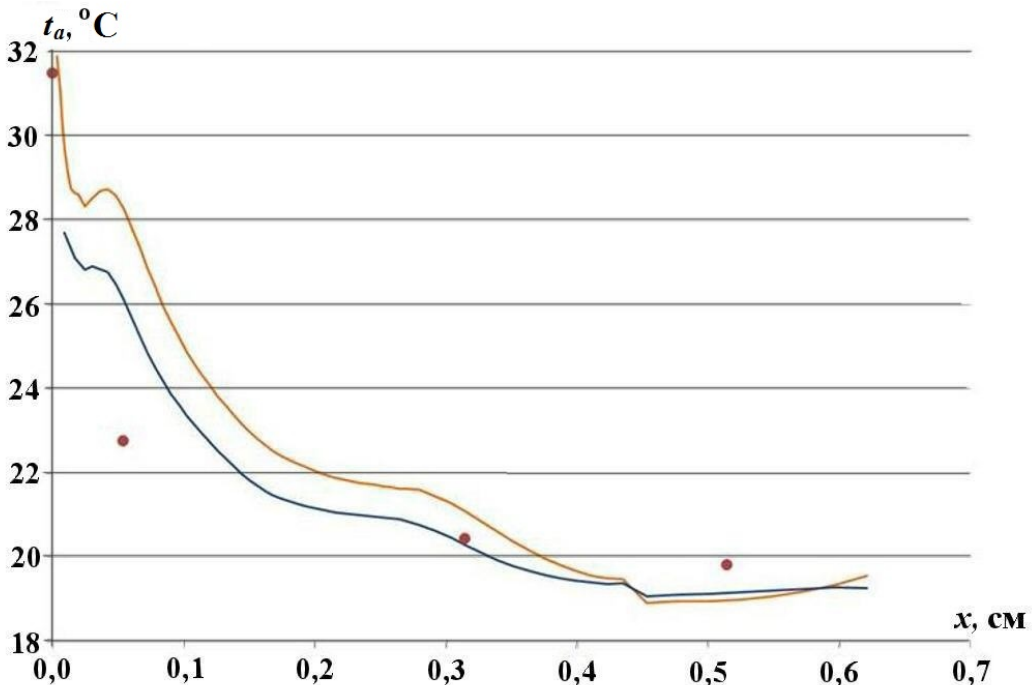
Рис. 7. Распределение температуры окружающего воздуха на вертикальной прямой, проходящей над плечом: ● — эксперимент; — — ЛОГОС без использования ТСМ; — — ЛОГОС с использованием ТСМ
