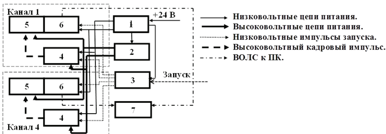
Рис. 1. Схема камеры СЭР-8: 1 – блок низковольтного питания, 2 – блок высоковольтного питания, 3 – модуль управления, 4 – генератор кадрового импульса, 5 – усилитель яркости (ЭОП), 6 – ПЗС-камера, 7 – персональный компьютер
