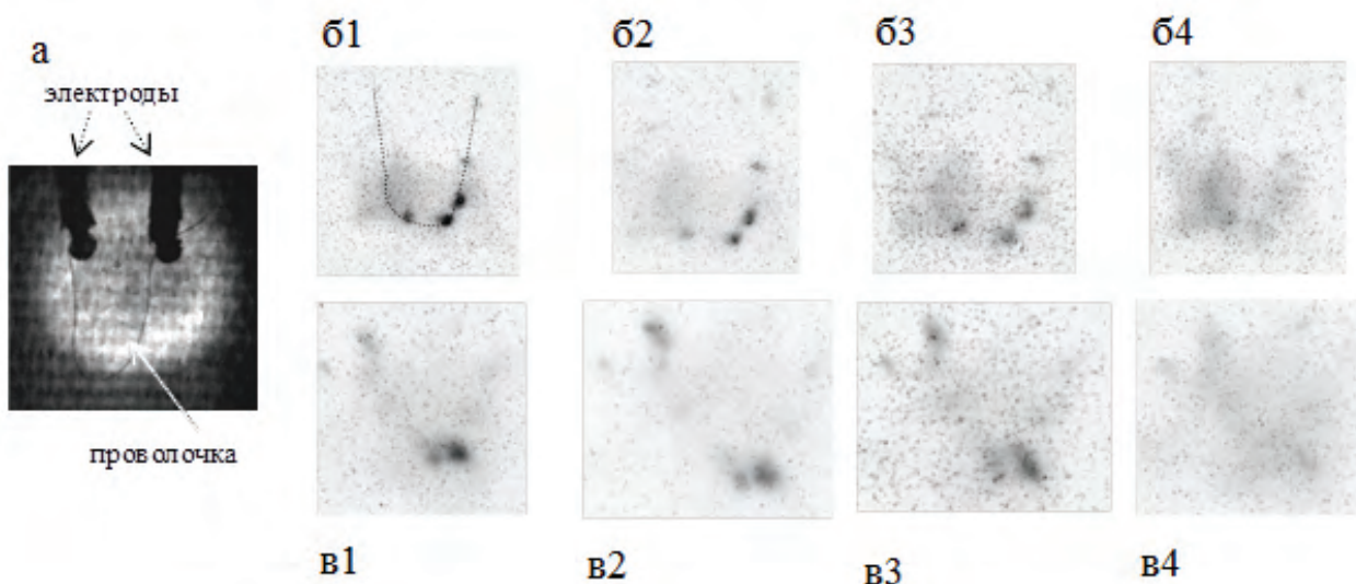
Рис. 4. Результаты регистрации 4-х кадровой камерой: а – настроечный кадр; б1-б4 – кадры регистрации разлета проволочки, снятые с задержкой 10мкс после срабатывания генератора; в1-в4 – кадры регистрации разлета проволочки, снятые с задержкой 30мкс после срабатывания генератора
