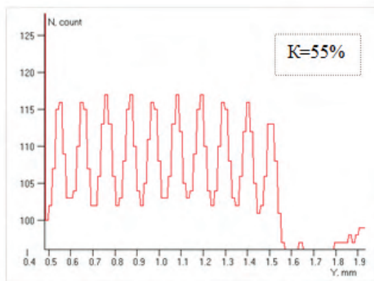
Рис. 3. Изображения миры № 3, при съемке с оптическим увеличением М5:1
