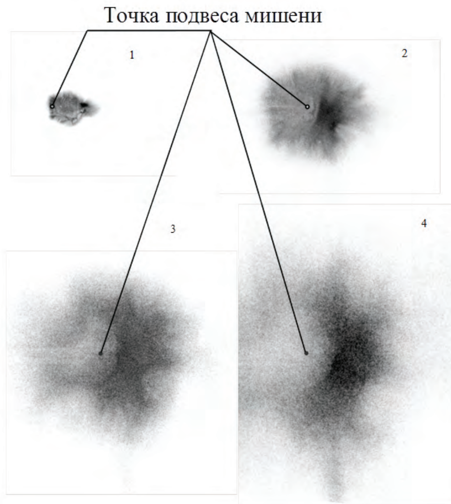
Рис. 6. Регистрация разлета сферы: 1 – 4 кадры регистрации
