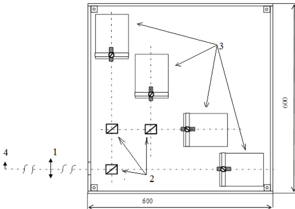
Рис. 2. Оптическая схема 4-х кадрового регистратора: 1 – объектив, 2 – светоделительные кубы, 3 – ЭОПы с ПЗС-камерами, 4 – тест-объект миры ГОИ № 4
