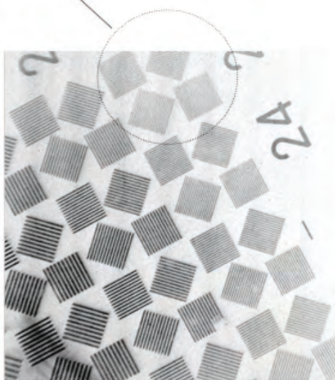
Рис. 3. Изображения миры № 3, при съемке с оптическим увеличением М5:1
