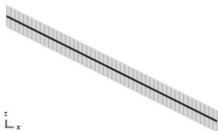
Рис. 4. Сетка со сгущением к поверхности раздела пластов
