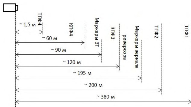
Рис. 4. Расстояния от электронной камеры ДСУ до маркеров
