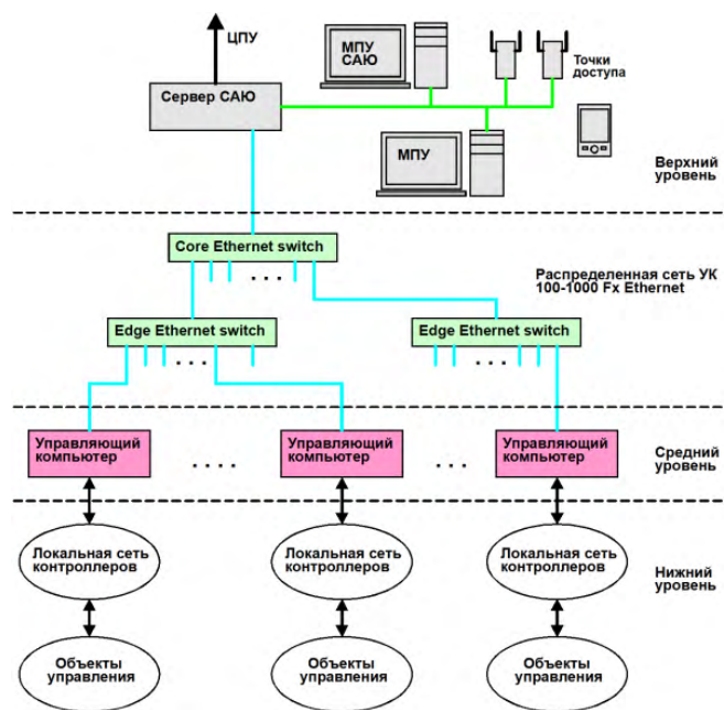
Рис. 1. Структурная схема управления САЮ
