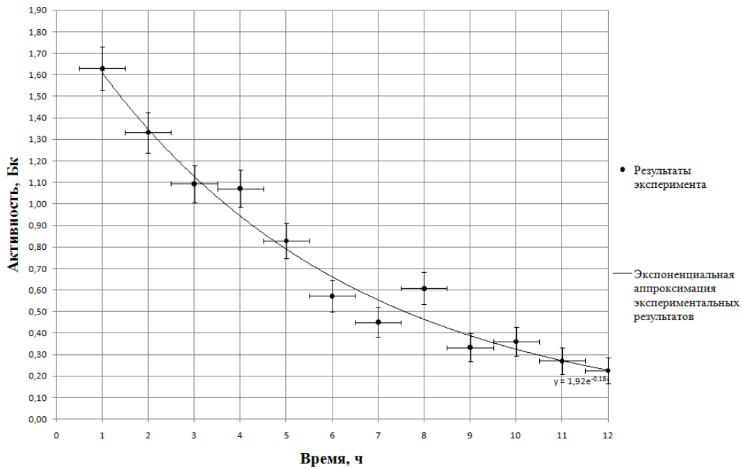
Рис. 2. Активность изомера в индиевом образце после эксперимента № 9
