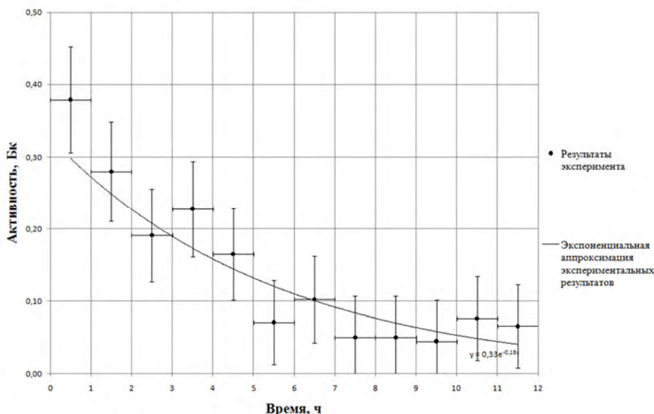
Рис. 1. Активность изомера в индиевом образце после эксперимента № 1
