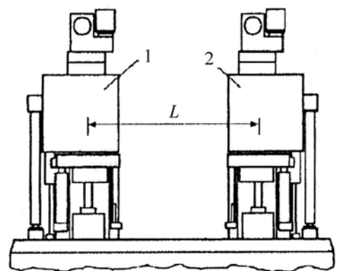
Рис. 7. Схема расположения на платформе подвижной (1) и неподвижной (2) АЗ реактора БАРС-6 ( L – расстояние между АЗ) [13]
