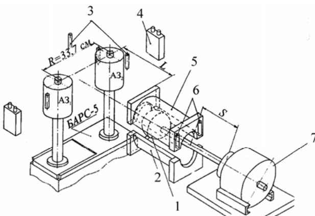
Рис. 6. Схема комплекса БАРС-5 + РУН [21]: 1 – капсула для образцов; 2, 5 – нижний и верхний блоки РУН; 3 – детекторы формы нейтронного импульса; 4, 6 – детекторы мощности БАРС-5 и РУН; 7 – загрузочное устройство; R – расстояние между осями АЗ БАРС-5; L – расстояние между БАРС-5 и РУН. Стенд умножителя не показан
