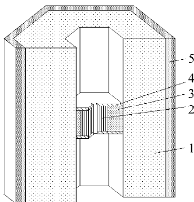
Рис. 4. Общий вид стенда УКС-1М [13]: 1 – внешняя размножающая зона; 2 – центральная размножающая зона; 3 – внутренний боковой отражатель; 4 – торцевой отражатель; 5 – наружный боковой отражатель
