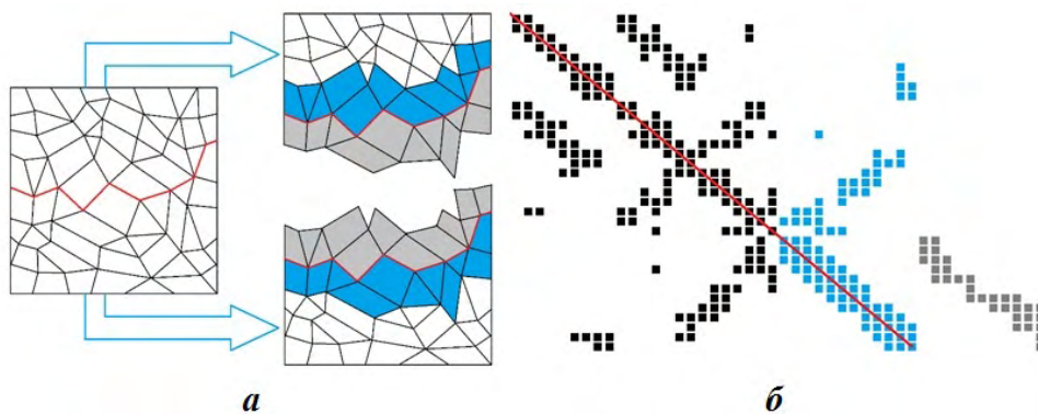
Рис. 2. Пример геометрической декомпозиции на две параобласти: a — сетки параобластей, б — портрет матрицы A для верхней параобласти
