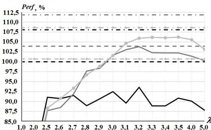
Рис. 7. Относительная производительность решения СЛАУ в зависимости от коэффициента балансировки при использовании четырех GPU на сетках с 19, 78, 312 млн ячеек: — — 19-HYBRID; — — 78-HYBRID; ●—●— 312-HYBRID; - - - 19-GPU; - - - 78-GPU; ●-●- 312-GPU; - · - · - 19-GPU+CPU; - · - · - 78-GPU+CPU; ●-·-●- 312-GPU+CPU
