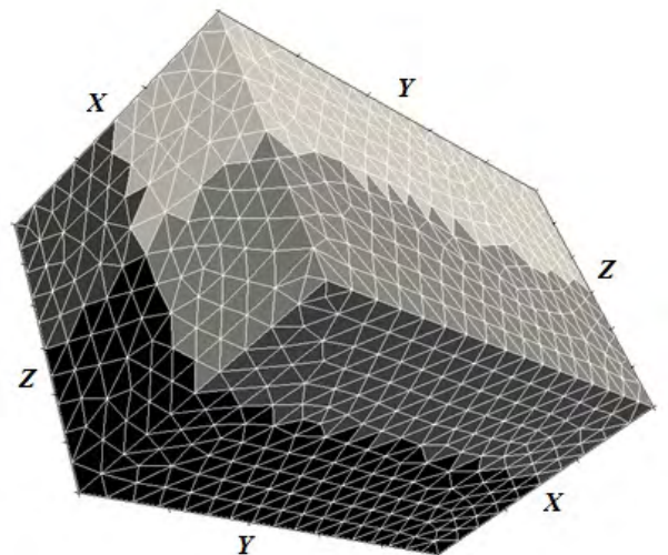
Рис. 5. Разбиение сетки А на четыре подобласти
