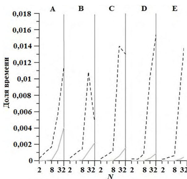
Рис. 9. Доля времени инициализации пересылок: --- — BS-метод; — — VJ-метод
