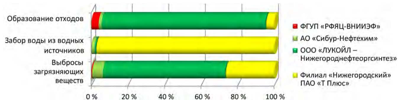
Рис. 7. Доля участия различных предприятий в общем объеме выбросов, сбросов и отходов
