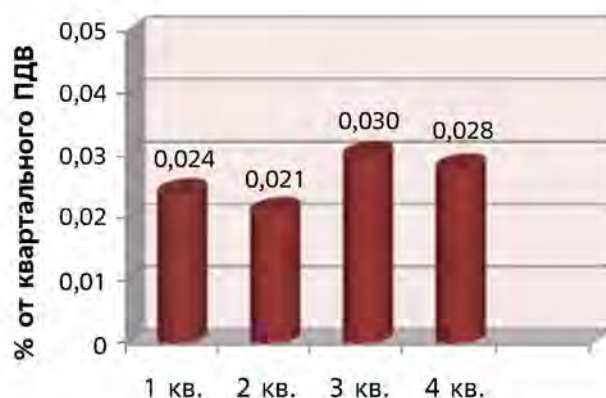
Рис. 4. Обобщенные данные по выбросам радионуклидов из источников ФГУП «РФЯЦ-ВНИИЭФ» в динамике за 2020 г.
