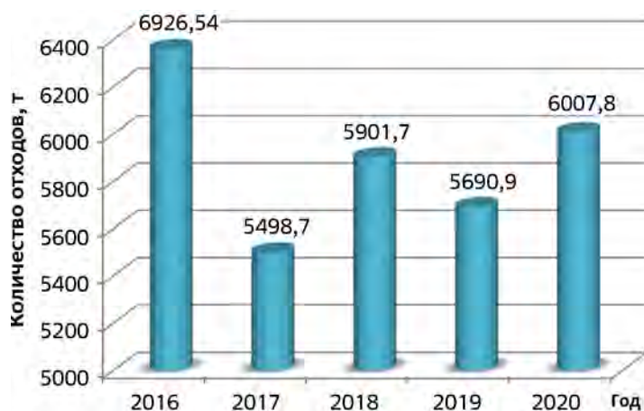
Рис. 5. Образование отходов в 2016–2020 гг.
