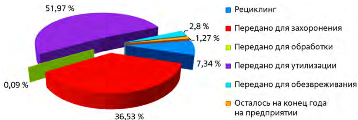
Рис. 6. Сведения об обращении с отходами производства и потребления в 2020 г.
