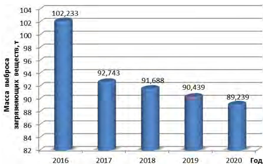
Рис. 2. Динамика массы выброса загрязняющих веществ (т/год) в атмосферный воздух за 2016–2020 гг.
