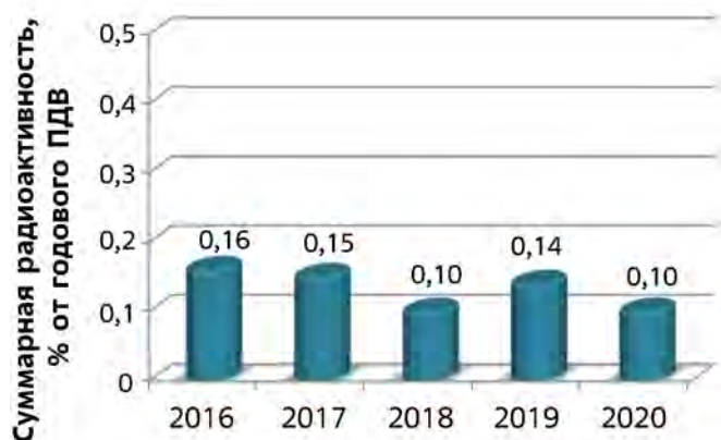
Рис. 3. Суммарные годовые фактические выбросы радионуклидов за 2016–2020 гг.
