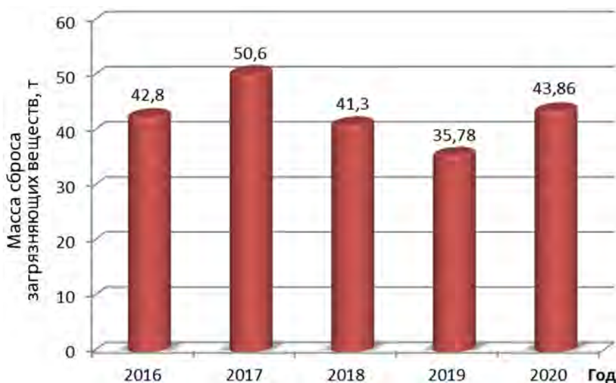
Рис. 1. Динамика сброса загрязняющих веществ с производственными сточными водами института (т/год) в водные объекты за период 2016–2020 гг.
