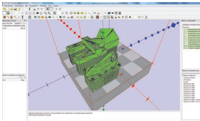
Рис. 7. Вид платформы с размещенными на ней деталями и построенными поддержками
