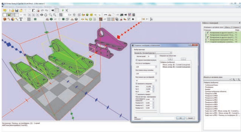
Рис. 1. Вид платформы с размещенными на ней деталями
