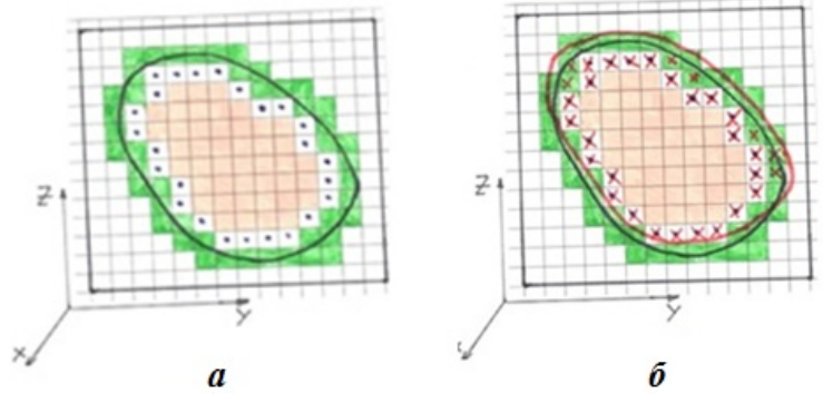
Рис. 7. Сечение поверхности и виды ячеек до ( а ) и после ( б ) ее передвижения
