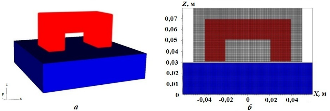
Рис. 1. Постановка задачи ( a ), расчетные области и сетки в сечении Y = 0 ( б )
