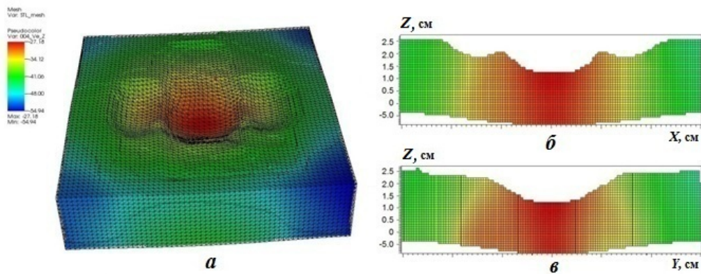
Рис. 14. Вид каверны в преграде при t=140 мкс: a — 3D изображение; b — сечение Y = 0 ; c — сечение X = 0 ; цветом показаны распределения вертикальной скорости
