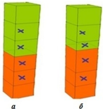
Рис. 9. Центральные ячейки локальной сетки до ( а ) и после ( б ) передвижения контактной поверхности и интегрирования
