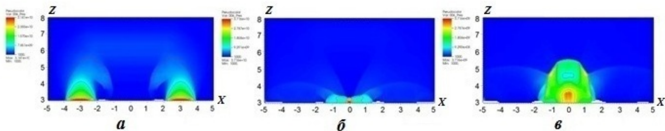
Рис. 10. Поля давлений (в Па) в газе в сечении Y = 0 : a - t = 4,9 мкс; b - t = 8 мкс; v - t = 12,2 мкс
