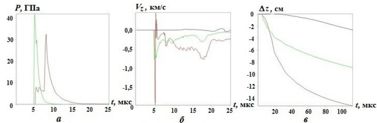
Рис. 13. Зависимости от времени давлений ( a ), скоростей ( b ) и перемещений ( v ) в лицевых точках преграды
