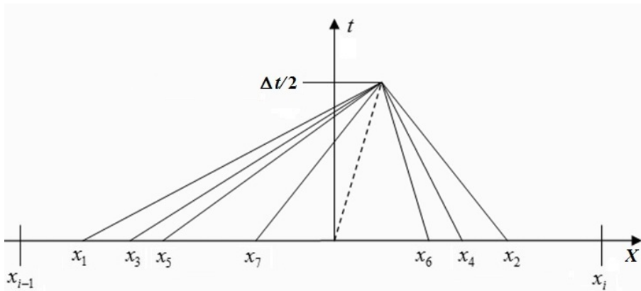
Рис. 5. Координаты проходящих инвариантов для грани интегрируемой ячейки на момент \Delta t/2
