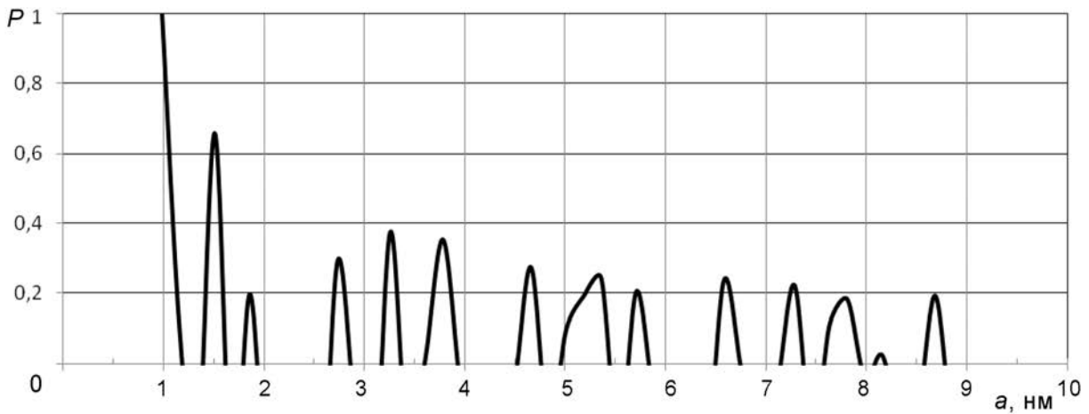
Рис. 1. Относительная плотность распределения наночастиц свинца по размерам в УВ внутри образца при T = 300 К (шаг расчетов равен 0,175 нм – атомный радиус [6], наибольший по величине P(a) локальный максимум после зародыша соответствует размеру 1,5 нм, расчет «оборван» на размере 10 нм)
