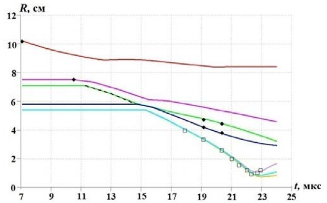
Рис. 4. (R, t) -диаграммы движения границ оболочек устройства 1: эксперимент [10, 12]: \square — результаты рентгенографирования; \blacklozenge — данные электроконтактной методики; — — — данные PDV; расчет: — — — внешняя граница оргстекла; — — — внешняя граница первого каскада; — — — внутренняя граница оболочки первого каскада; — — — внешняя граница второго каскада; — — —, — — —, — — — — внутренние границы оболочки второго каскада для \varphi = 0, 30, 90^\circ соответственно
