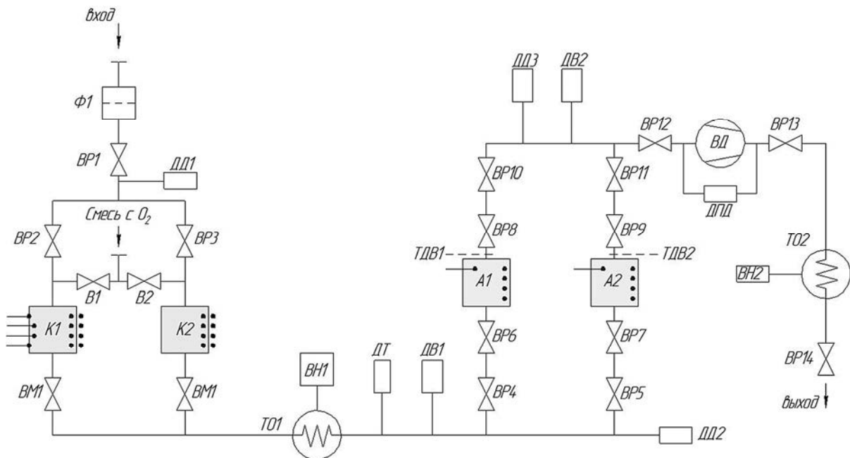
Рис. 1. Принципиальная газовакуумная схема.
