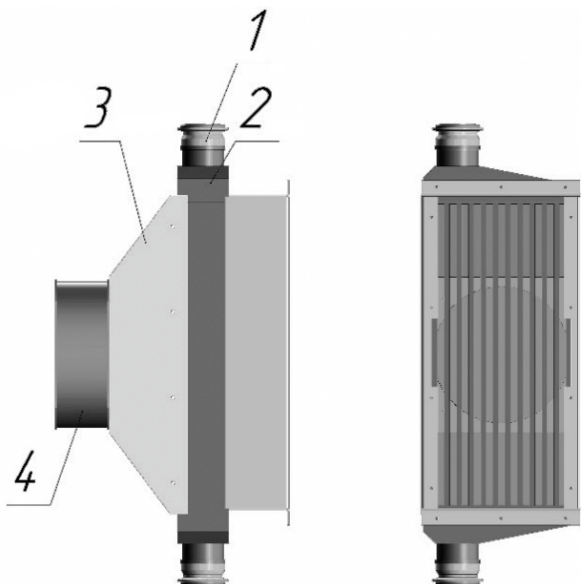
Рис. 6. Основные составные части теплообменника: 1 – входной фланец; 2 – корпус; 3 – кожух; 4 – вентилятор
