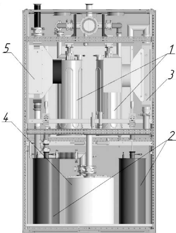
Рис. 2. Основные составные части установки очистки газовой среды от трития: 1 – конвертер; 2 – адсорбер; 3 – теплообменник; 4 – воздуходувка; 5 – выходной теплообменник
