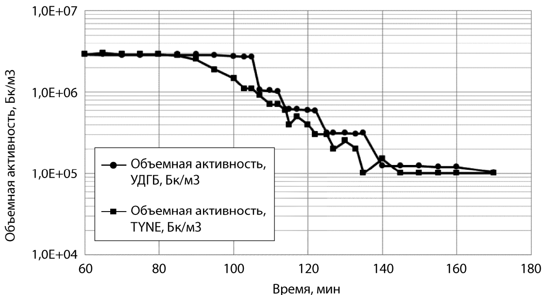
Рис. 7. Результаты измерений ОА газовой смеси двумя различными радиометрами на выходе из газоочистки в ходе процесса очистки ресивера от трития
