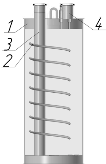
Рис. 4. Основные составные части многогазового адсорбера: 1 – камера герметичная; 2 – нагреватель; 3 – входной трубопровод; 4 – выходной патрубок
