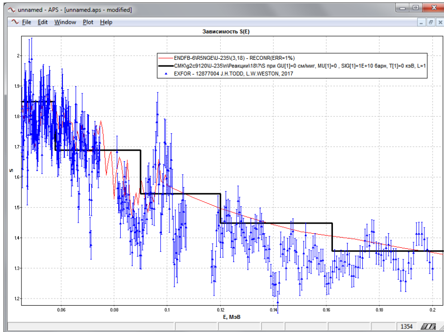
Рис. 13. Пример графического отображения сечения деления ^{235}\text{U} из разных источников: \blacktriangle – экспериментальные данные EXFOR, — — — о цененные данные ENDF/B-6, — — — групповые данные БД GROUND2
