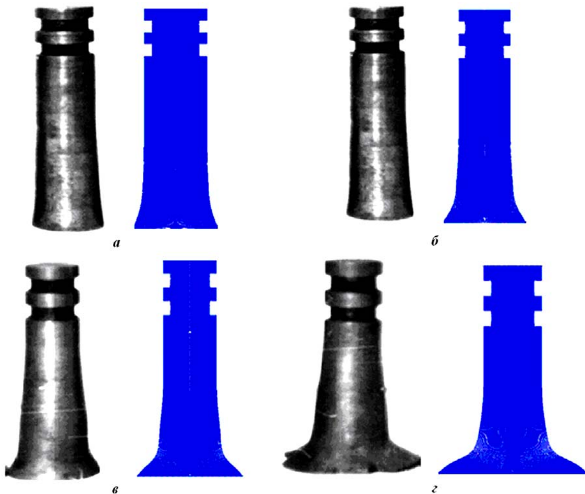
Рис. 2. Конечная форма стержня из стали: а — v_0 = 0,120 км/с; б — v_0 = 0,170 км/с; в — v_0 = 0,235 км/с; г — v_0 = 0,310 км/с; слева — эксперимент; справа — расчет по методике ИНЧ-М
