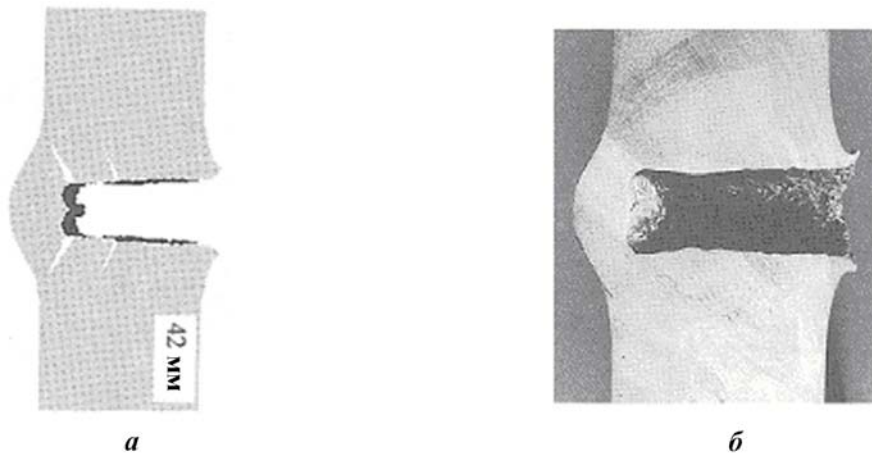
Рис. 8. Формы остаточного кратера, толщина мишени 4,2 см, t = 120 мс: a — расчет OTI*HULL; б — эксперимент
