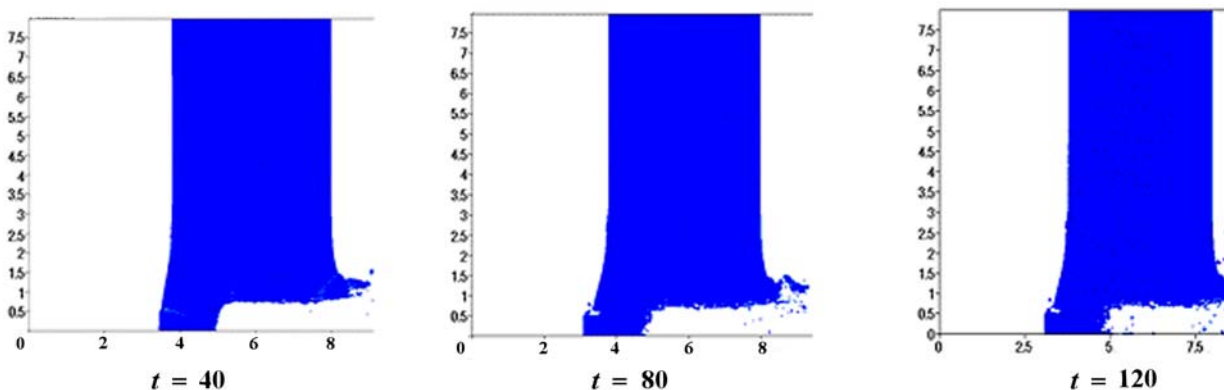
Рис. 6. Динамика пробивания мишени ПЭ толщиной 4,2 см. Расчет ИНЧ-М
