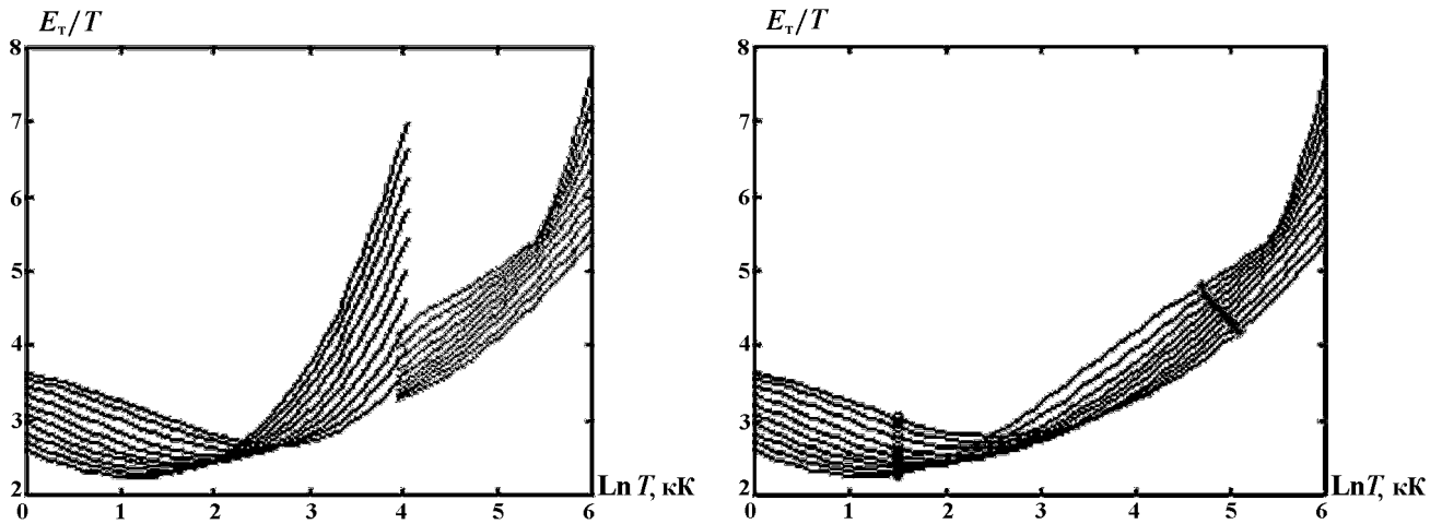
Рис. 4. Изохоры функции \varepsilon = E_\tau/T до (слева) и после (справа) сшивки
