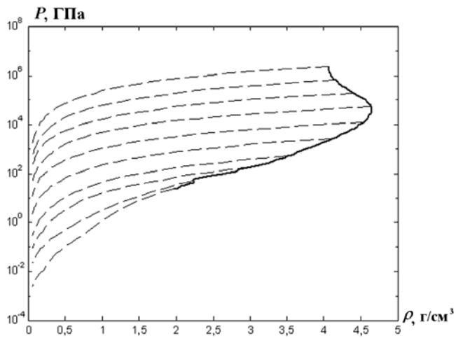
Рис. 5. Ударная адиабата (—) и изэнтропы разгрузки (- - -) воды
