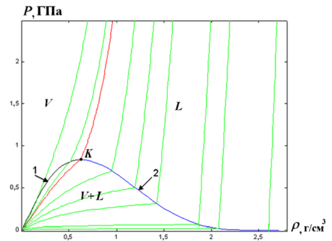
Рис. 1. Фазовая диаграмма и изэнтропы алюминия: L — жидкость; V — пар; V + L — равновесная смесь пара и жидкости; 1 — линия конденсации; 2 — линия испарения; K — критическая точка
