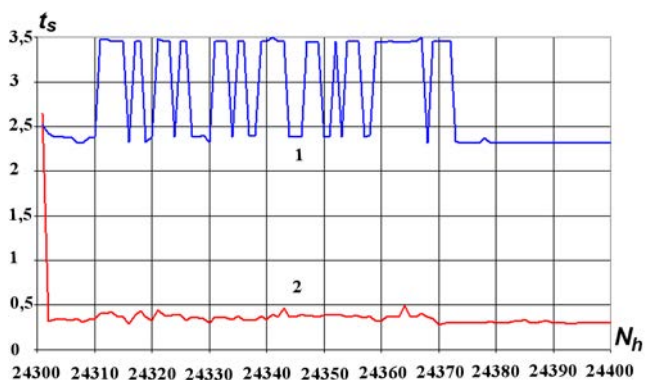
Рис. 9. Задача 3. График зависимости времени решения линейной системы на одном временном шаге от номера шага: 1 — в штатном режиме; 2 — с адаптивным выбором решателя
