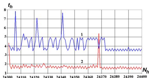
Рис. 7. Задача 2. Изменение сложности линейных систем в процессе одного из временных шагов решения уравнения теплопроводности
