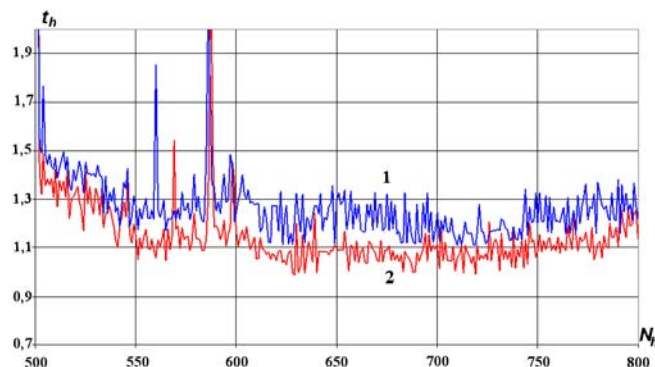
Рис. 5. Задача 2. График зависимости полного времени счета одного временного шага от номера шага: 1 — в штатном режиме; 2 — с адаптивным выбором решателя
