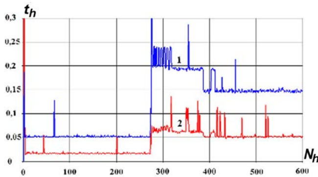
Рис. 11. Задача 4. График зависимости времени решения линейной системы на одном временном шаге от номера шага: 1 — в штатном режиме; 2 — с адаптивным выбором решателя
