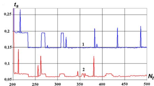
Рис. 2. Задача 1. График зависимости полного времени счета одного временного шага от номера шага: 1 — в штатном режиме; 2 — с адаптивным выбором решателя
