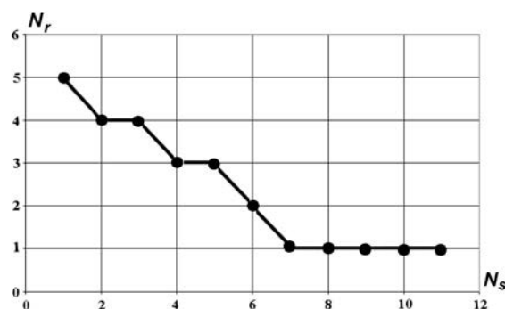
Рис. 7. Задача 2. Изменение сложности линейных систем в процессе одного из временных шагов решения уравнения теплопроводности
