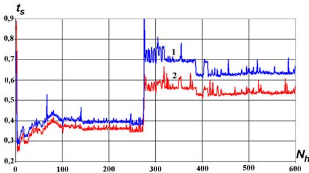
Рис. 10. Задача 4. График зависимости полного времени счета одного временного шага от номера шага: 1 — в штатном режиме; 2 — с адаптивным выбором решателя
