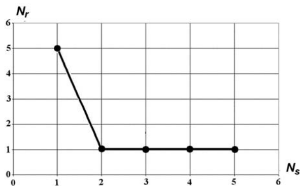
Рис. 4. Задача 1. Динамика изменения сложности линейных систем в процессе одного из временных шагов решения уравнения теплопроводности
