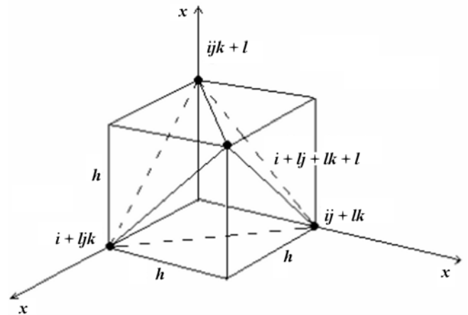
Рис. 5. Элемент ажурной схемы — центральный тетраэдр внутри куба (остальные четыре тетраэдра в расчетах не участвуют)
