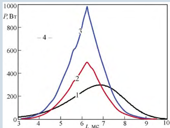
Параллельное объединение двух лазерных каналов на установке ЛУНА-2М: импульс реактора ВИР-2М (1); одинарный лазерный канал (2); двойной канал (3)
