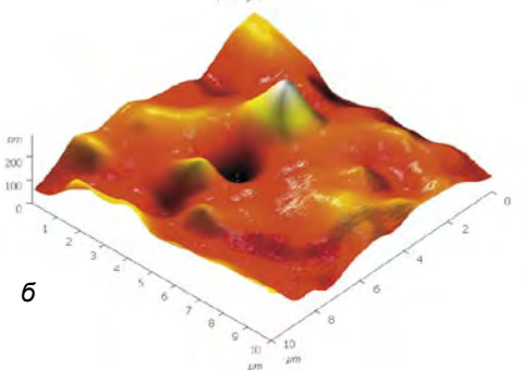
Поверхность полимеров, модифицированных методом молекулярного наслаивания (а) и углеродными наноструктурами (б)
