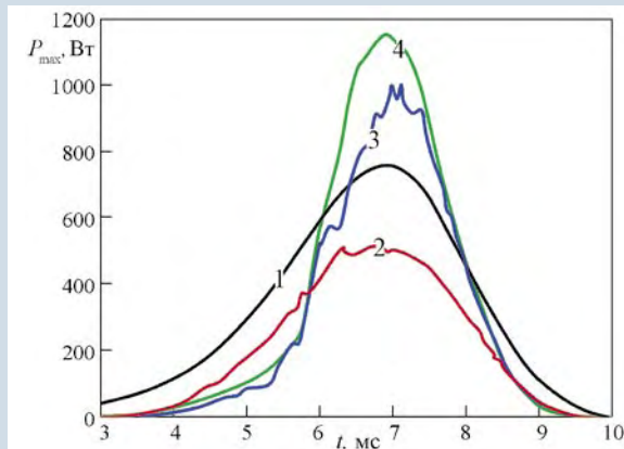
Последовательное объединение двух лазерных каналов на установке ЛУНА-2М: импульс реактора ВИР-2М (1); одинарный лазерный канал (2); двойной канал (3); расчетная мощность генерации двойного канала для коэффициента отражения поворотных зеркал 100 % (4)
