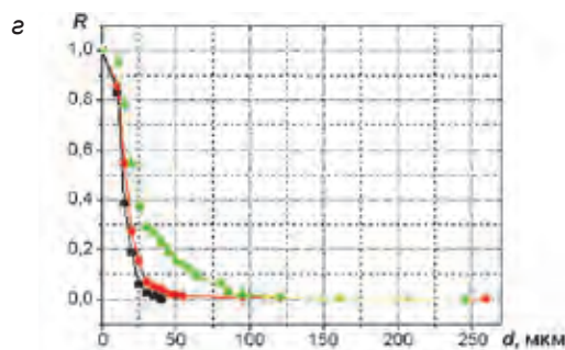
Видеокадры частиц свинца (а – в) и относительное распределение выброшенных частиц по размерам (г): ■ – Rz5; ● – Rz20; ▲ – Rz80
