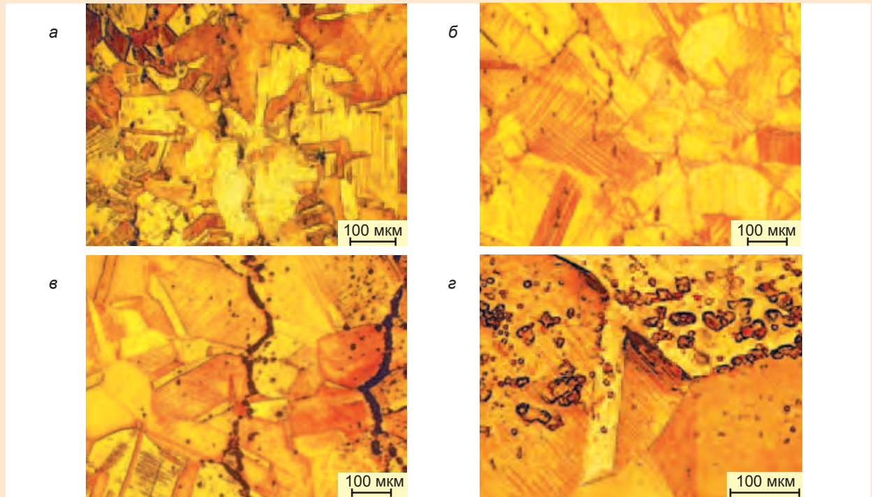
Микроструктура образцов после эксперимента по определению поврежденности. Масштаб: а – 1:1; б – 1:2; в – 1:4; г – 1:8
