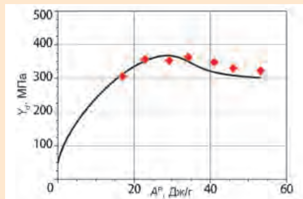
Расчетная (—) и экспериментальная (◆) зависимости предела текучести от работы ударно-волнового пластического деформирования меди до давлений P = 70 ГПа
