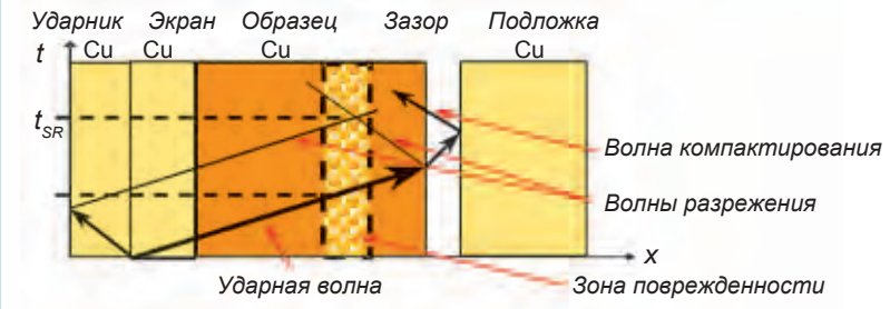
Схема эксперимента по определению поврежденности
