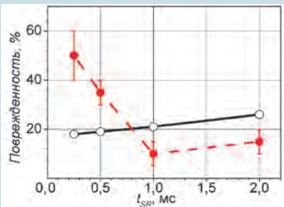
Зависимость максимальной поврежденности от времени прихода откольного импульса нагружения ~35 ГПа: ○ – расчет NAG; ● – эксперимент
