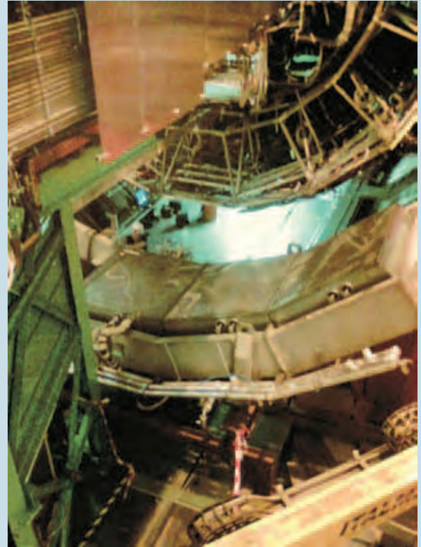
Установка последнего модуля спектрометра PHOS в опорную структуру (фото слева) и трехмодульный спектрометр перед его установкой на рабочую позицию в магнит (фото справа)
