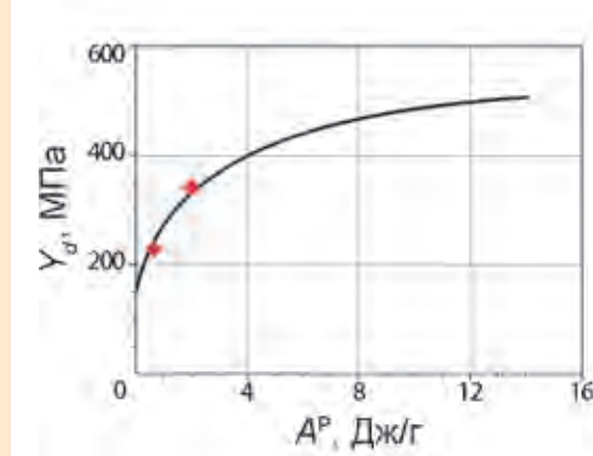
Зависимость предела текучести тантала от работы пластического деформирования при статическом (—) и ударно-волновом (◆) деформировании
