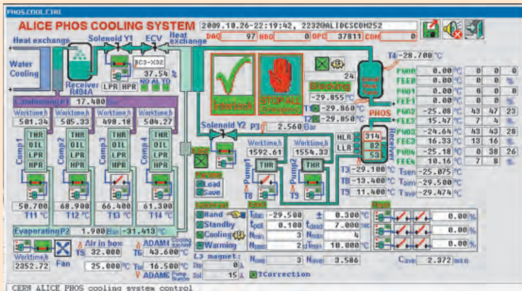
Панель управления системы охлаждения матрицы кристаллов
