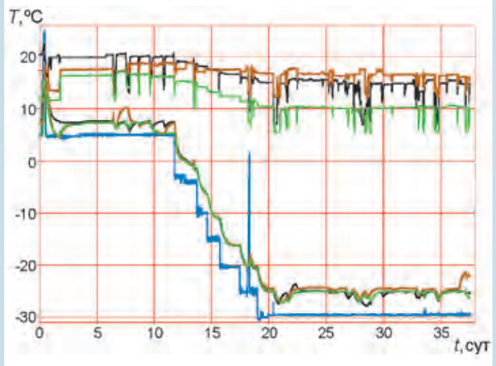
Графики температуры теплоносителя, массива кристаллов PbWO_4 и элементов электроники одного из модулей спектрометра PHOS (с 01.10.2009 г., 0 ч 0 мин)
