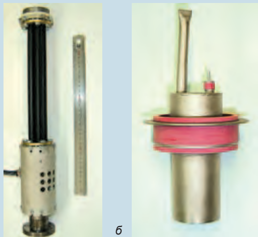
ВЧ-генераторы: а – генератор на 220 МГц с импульсной мощностью 8 МВт; б – отпаянная камера портативного ВЧ-генератора
