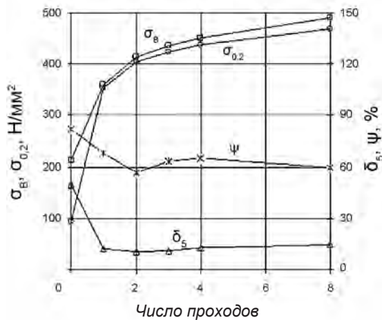
Зависимость механических свойств меди М1 от числа проходов
