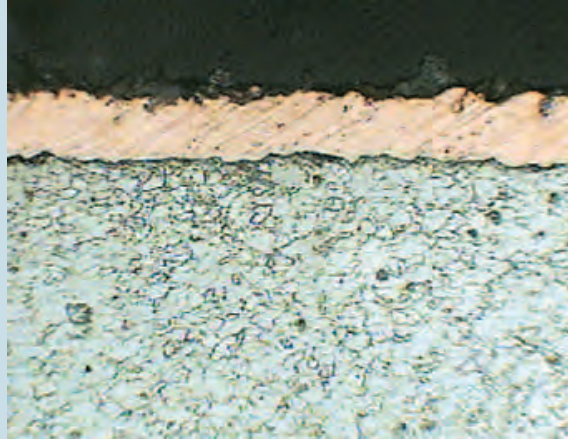
Гальваническое покрытие меди на магнитомягком сплаве 27КХ
