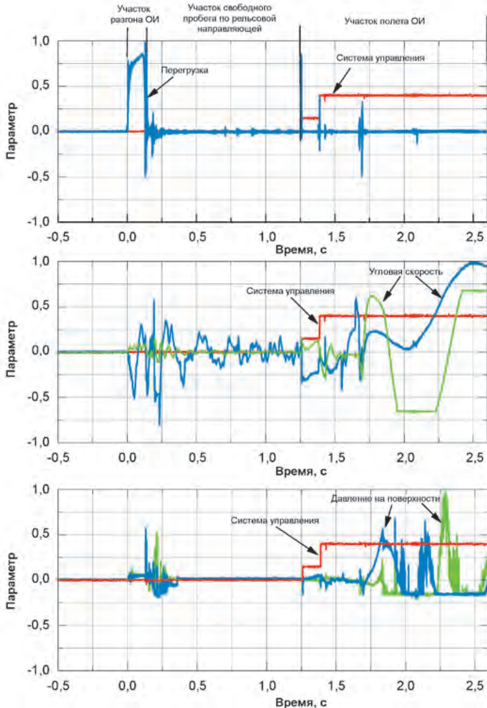
Изменение параметров движения в опыте с разгоном изделия по рельсовым направляющим ракетного трека
